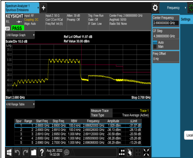
Band41-5MHz-16QAM-41565-1RB#24
