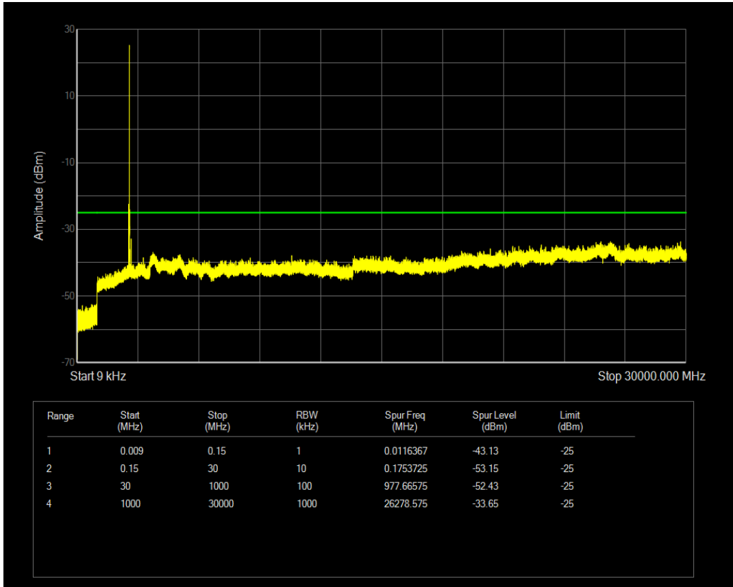
n41(2535-2655) SCS=15kHz DFT_QPSK BW=10MHz Channel=519000 RB=1@51
