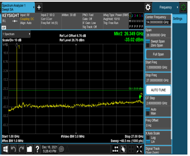
Band41-5MHz-16QAM-40640-1RB#0-Range2:1000~27000MHz
