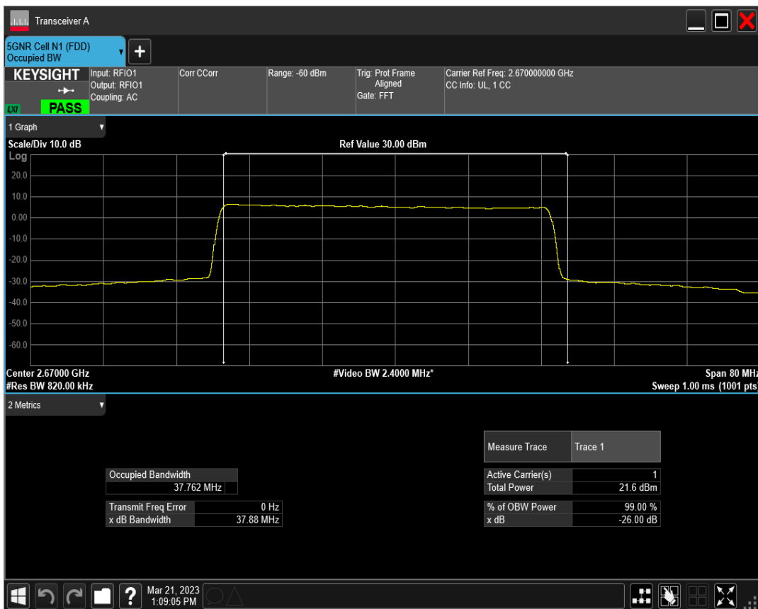
n41 SCS=30kHz CP_QPSK BW=40MHz Channel=534000 RB=106@0
