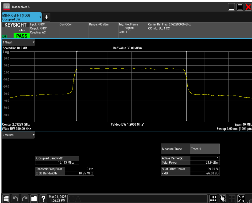
n41 SCS=30kHz CP_QPSK BW=20MHz Channel=518598 RB=51@0
