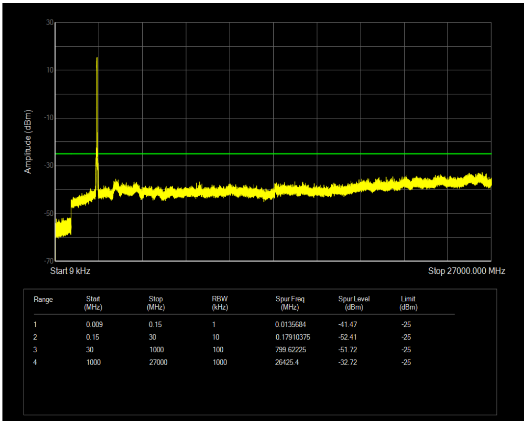
n38 SCS=15kHz DFT_QPSK BW=40MHz Channel=520000 RB=1@0
