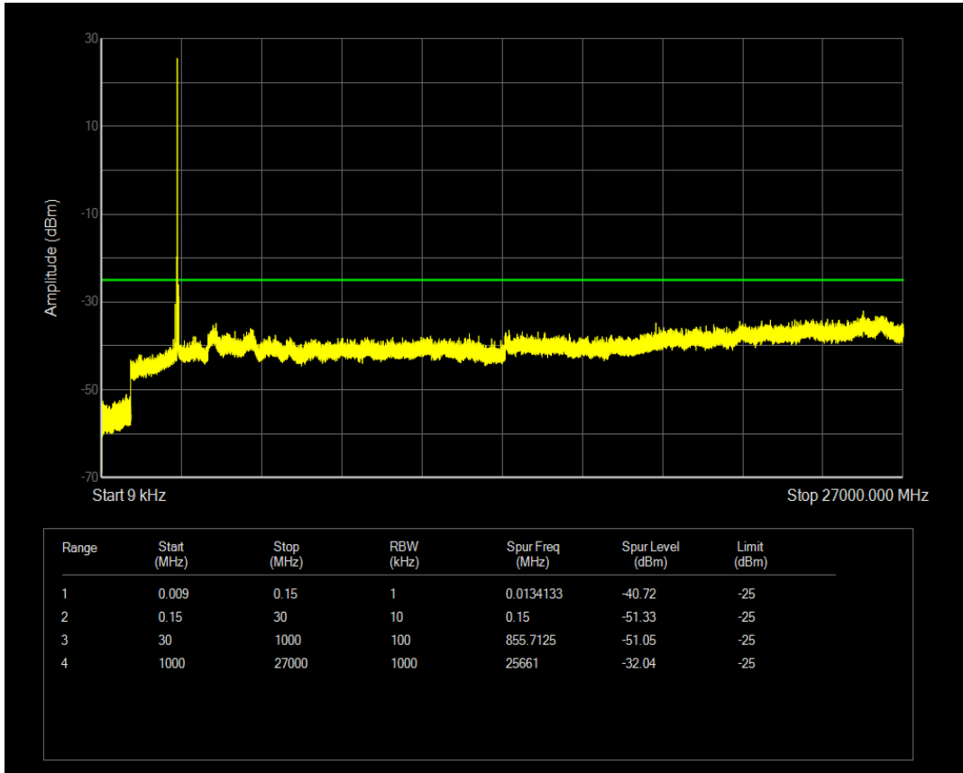
n38 SCS=15kHz DFT_QPSK BW=40MHz Channel=518000 RB=1@215
