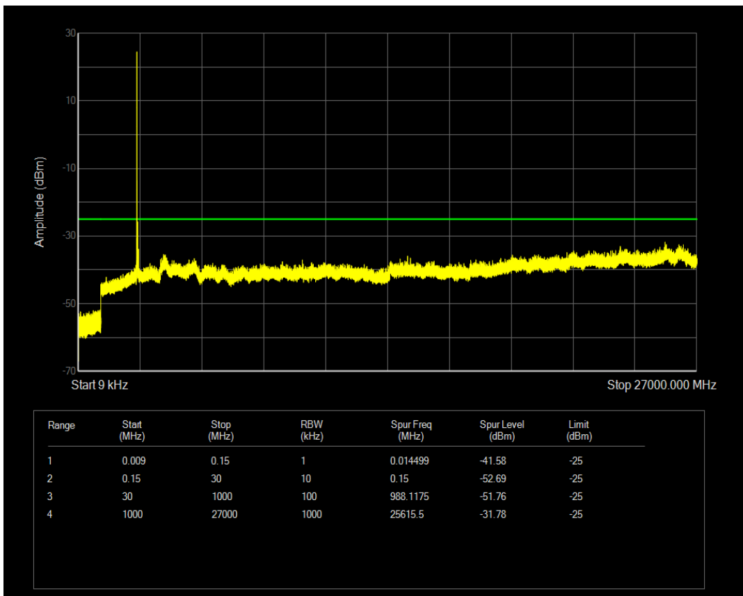
n38 SCS=15kHz DFT_QPSK BW=40MHz Channel=519000 RB=1@215
