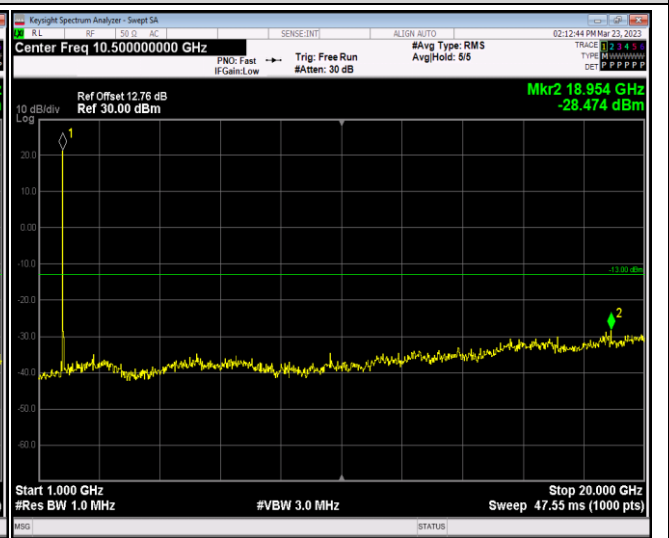
Band66-20MHz-QPSK-132572-1RB#0-Range2:1000~ 20000MHz
