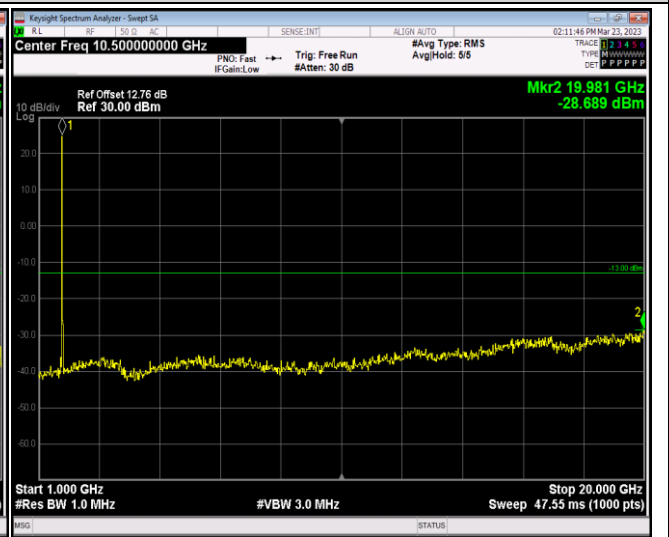
Band66-20MHz-QPSK-132572-1RB#0-Range2:1000~ 20000MHz
