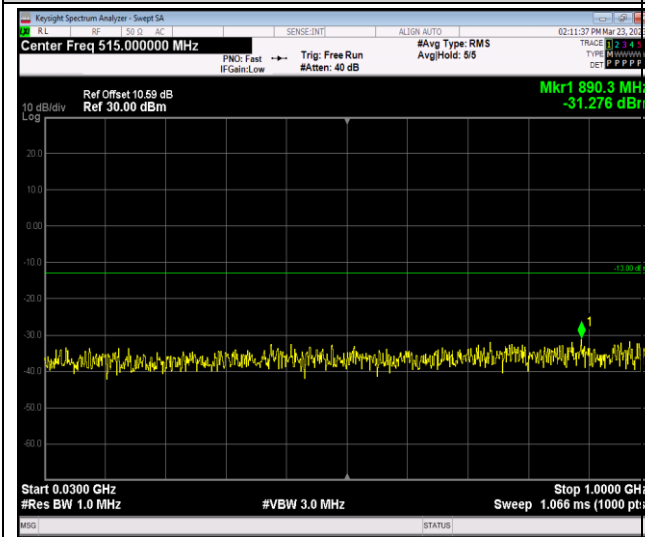
Band66-20MHz-QPSK-132572-1RB#0-Range1:30 ~1000MHz
