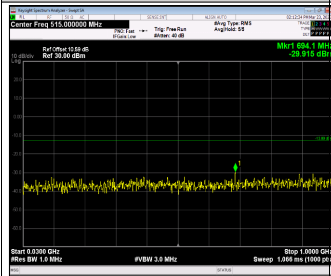
Band66-20MHz-QPSK-132572-1RB#0-Range1:30 ~1000MHz
