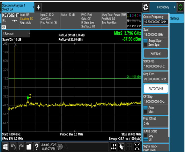
Band2-20MHz-QPSK-18700-1RB#0-Range2:1000~20000MHz
