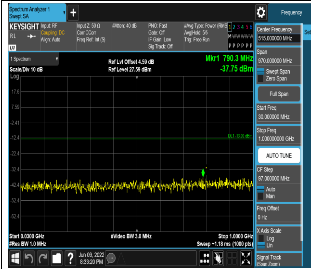
Band2-20MHz-QPSK-18700-1RB#0-Range1:30~1000MHz
