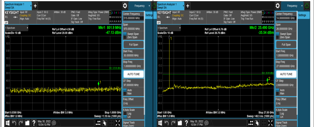
Band7-20MHz-QPSK-20850-1RB#0-Range1:30~1 000MHz Band7-20MHz-QPSK-20850-1RB#0-Range2:1000~27 000MHz
