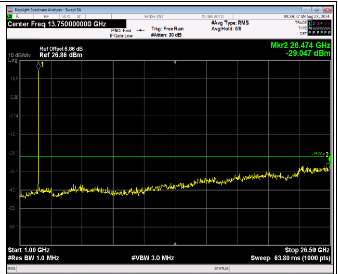
Band7-20MHz-16QAM-21350-1RB#0-Range2:1000~26500MHz
