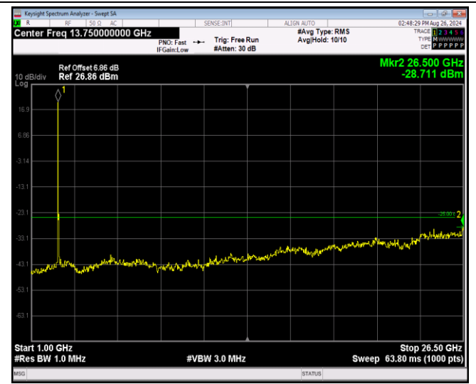
Band41-20MHz-QPSK-41140-1RB#0-Range2:1000~2 6500MHz
