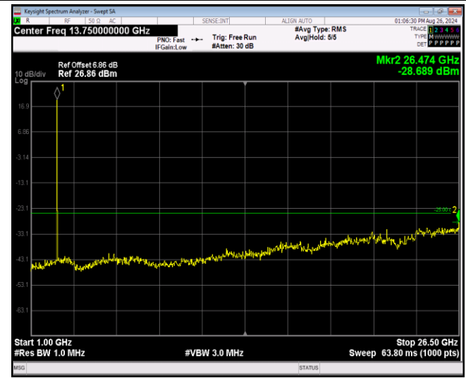
Band7-5MHz-16QAM-21425-1RB#0-Range2:1000~26 500MHz
