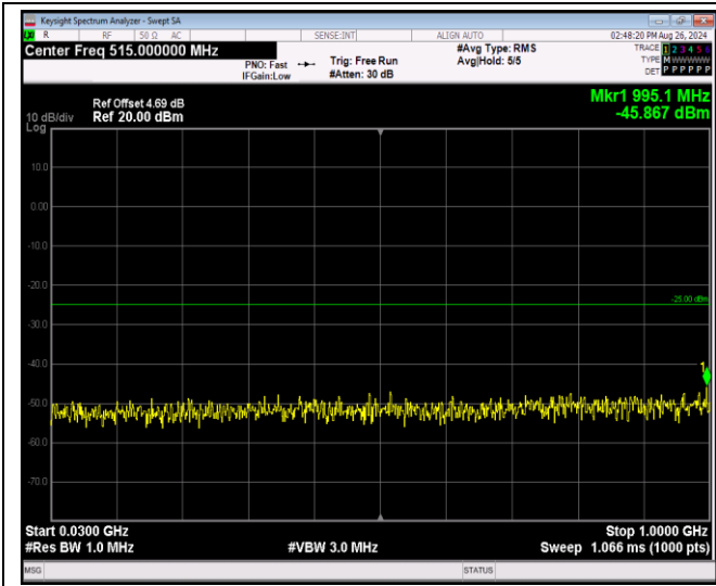
Band41-20MHz-QPSK-41140-1RB#0-Range1:30~100 0MHz
