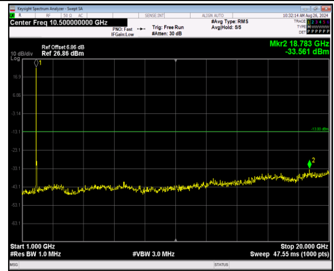
Band2-20MHz-16QAM-19100-1RB#0-Range2:1000~2 0000MHz
