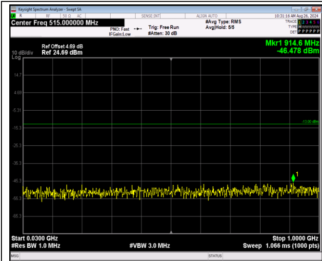
Band2-20MHz-16QAM-18900-1RB#0-Range1:30~100 OMHz
