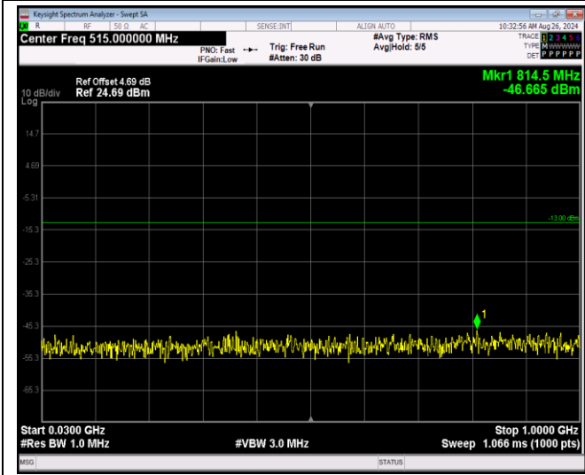
Band2-20MHz-16QAM-19100-1RB#0-Range1:30~100 OMHz
