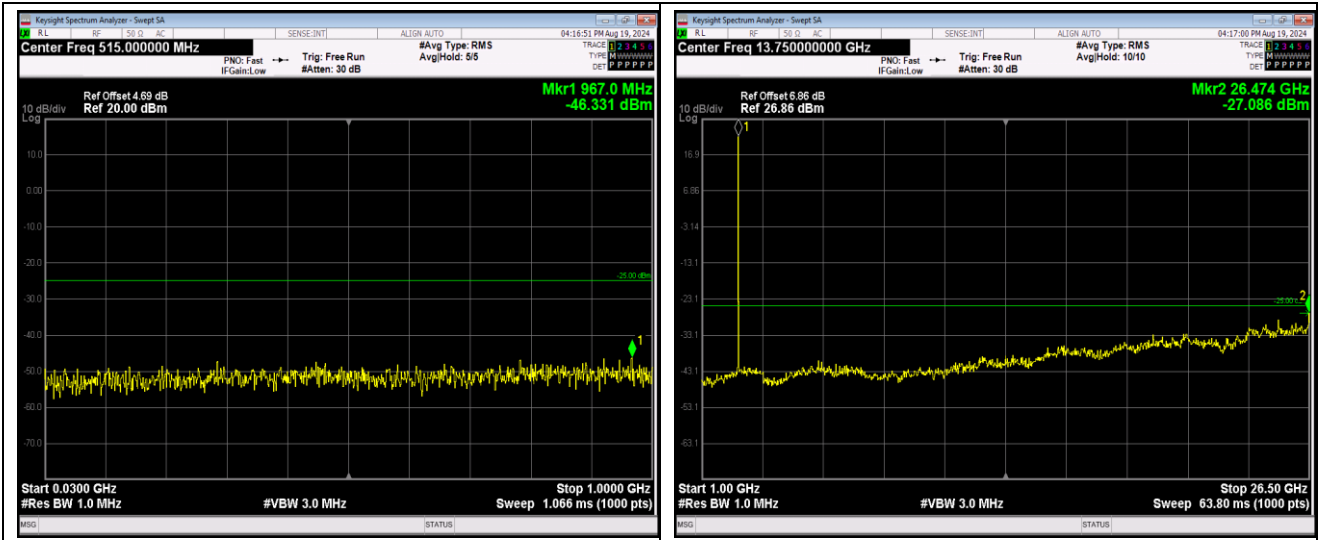
Band41-5MHz-QPSK-40640-1RB#0-Range1:30~100 0MHz
