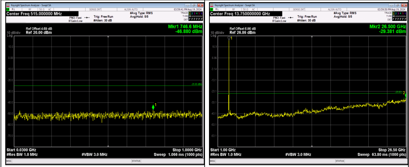
Band7-20MHz-QPSK-21100-1RB#0-Range1:30~100 0MHz
