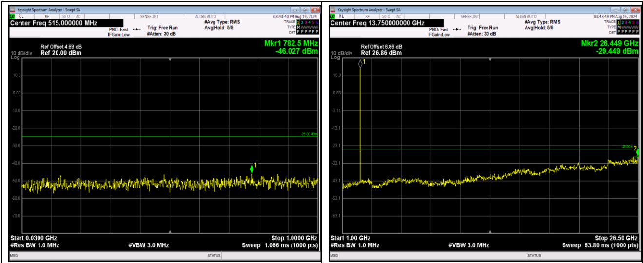
Band7-20MHz-QPSK-20850-1RB#0-Range1:30~100 0MHz
