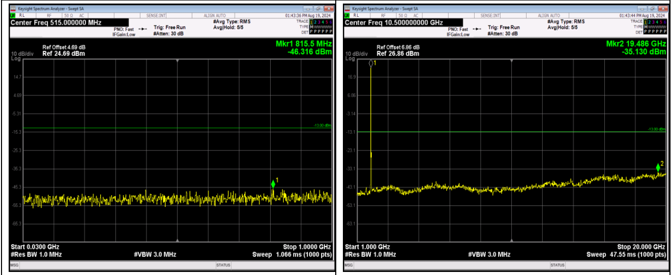
Band2-20MHz-QPSK-18700-1RB#0-Range1:30~1000MHz
