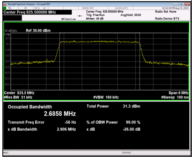
Band5-3MHz-QPSK-20635-15RB#0
