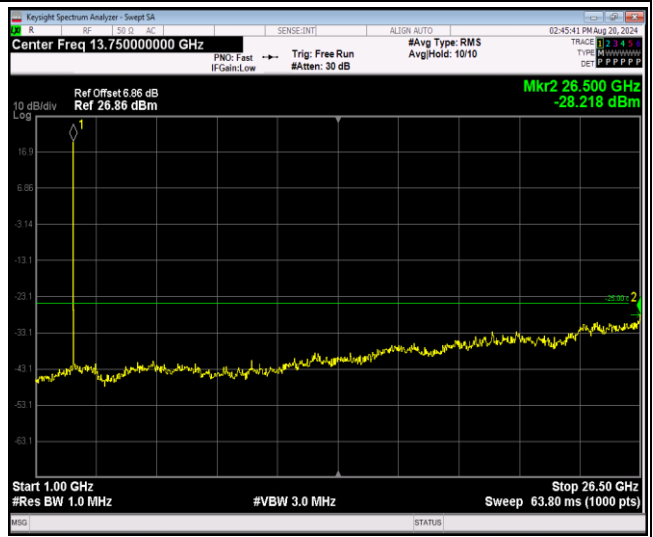
Band41-5MHz-QPSK-41215-1RB#0-Range2:1000~2 6500MHz
