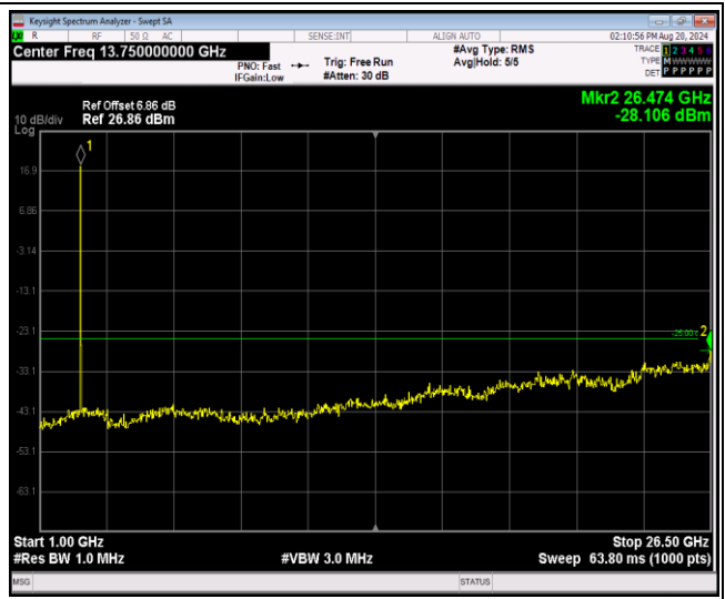
Band7-20MHz-QPSK-20850-1RB#0-Range2:1000~2 6500MHz
