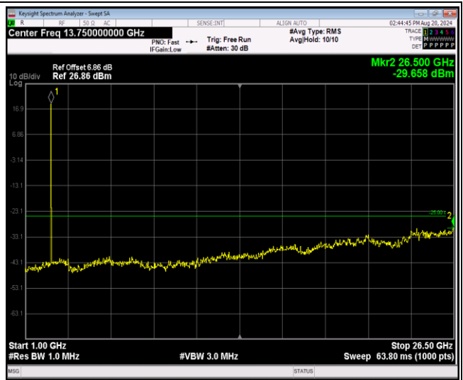
Band41-5MHz-QPSK-40640-1RB#0-Range2:1000~2 6500MHz
