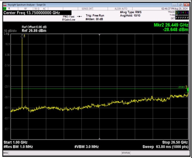
Band41-5MHz-QPSK-41215-1RB#0-Range2:1000~2 6500MHz
