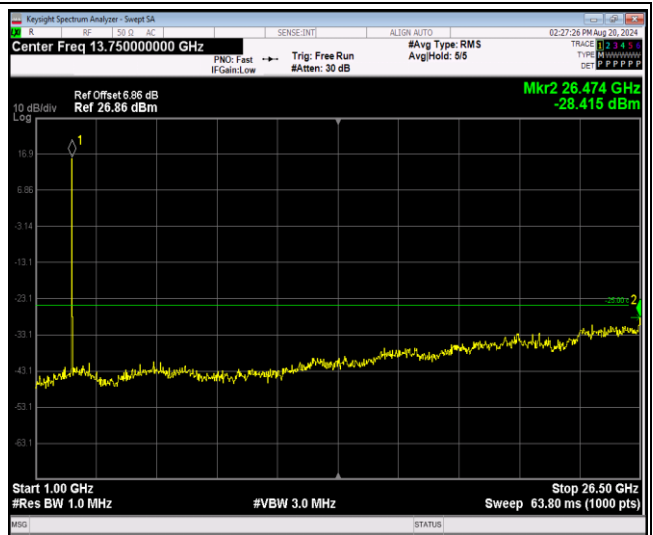
Band7-20MHz-16QAM-21350-1RB#0-Range2:1000~26500MHz
