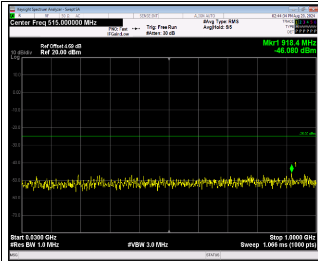
Band41-5MHz-QPSK-40640-1RB#0-Range1:30~100 0MHz
