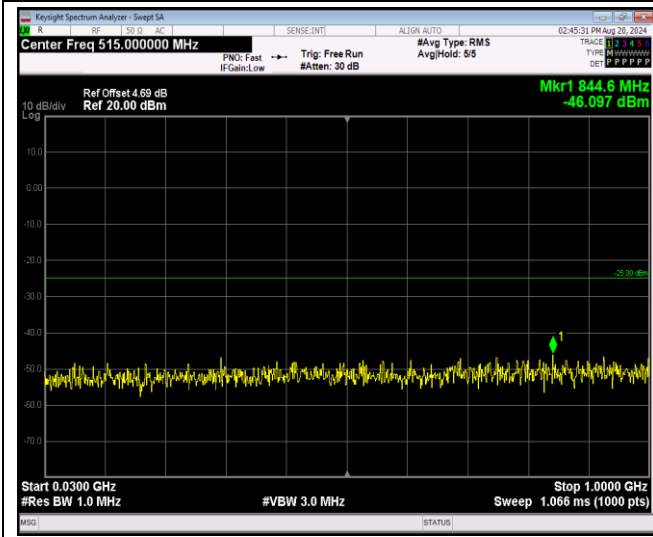
Band41-5MHz-QPSK-41215-1RB#0-Range1:30~100 0MHz
