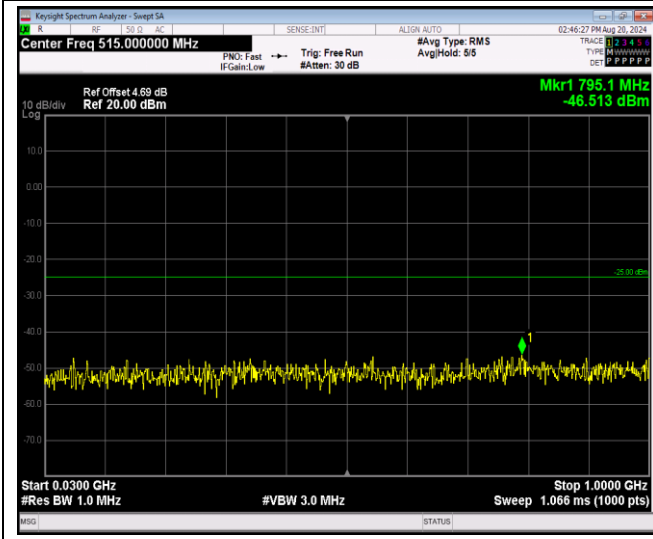
Band41-5MHz-QPSK-41215-1RB#0-Range1:30~100 0MHz
