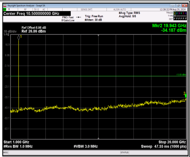
Band4-1.4MHz-QPSK-19957-1RB#0-Range2:1000~20000MHz
