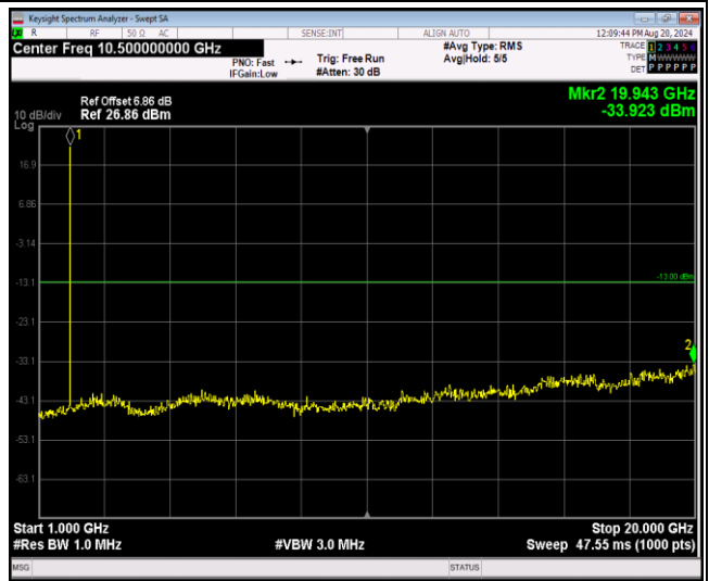
Band2-20MHz-QPSK-18700-1RB#0-Range2:1000~20000MHz
