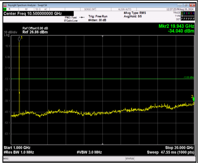
Band2-20MHz-16QAM-19100-1RB#0-Range2:1000~20000MHz
