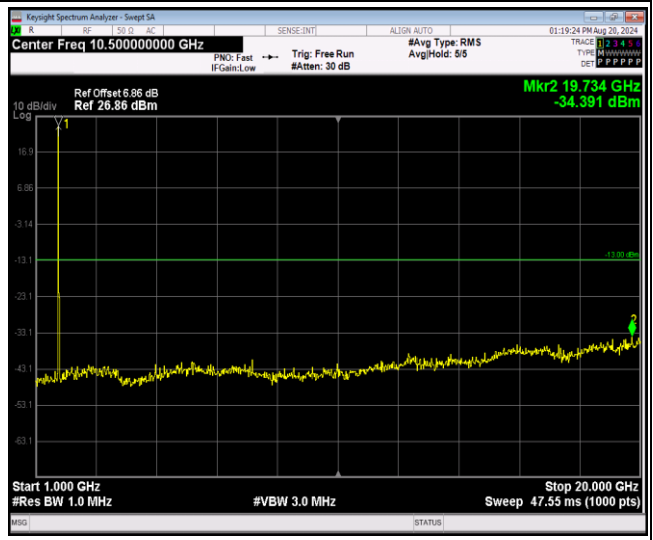
Band4-20MHz-QPSK-20300-1RB#0-Range2:1000~2 0000MHz
