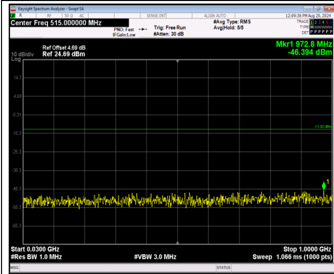
Band2-20MHz-QPSK-18700-1RB#0-Range1:30~1000MHz
