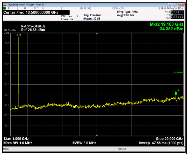
Band2-20MHz-16QAM-19100-1RB#0-Range2:1000~20000MHz
