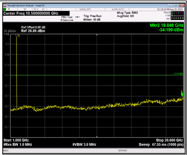
Band4-20MHz-QPSK-20175-1RB#0-Range2:1000~2 0000MHz
