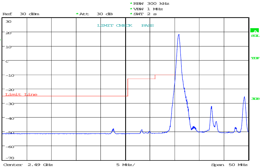
BW15MHz-2507.5MHz,Q16-1RB_MID@Pass
