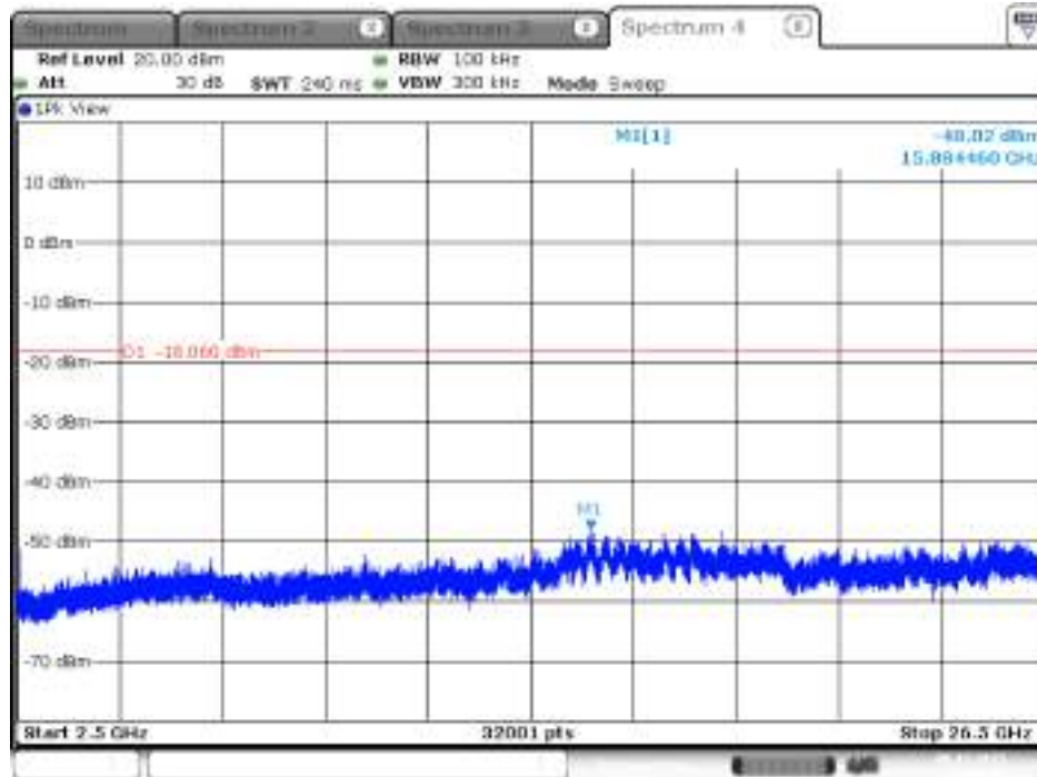
Plot on Configuration IEEE 802.11b / 2412 MHz / 2500MHz~26500MHz (down 30dBc) / Chain 2
