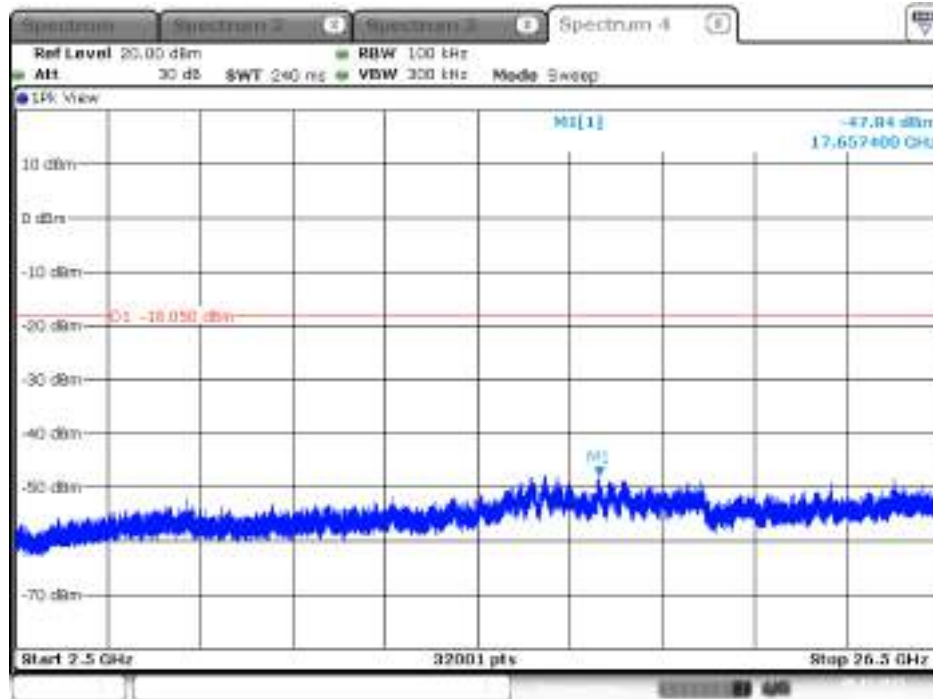
Plot on Configuration IEEE 802.11b / 2412 MHz / 2500MHz~26500MHz (down 30dBc) / Chain 1
