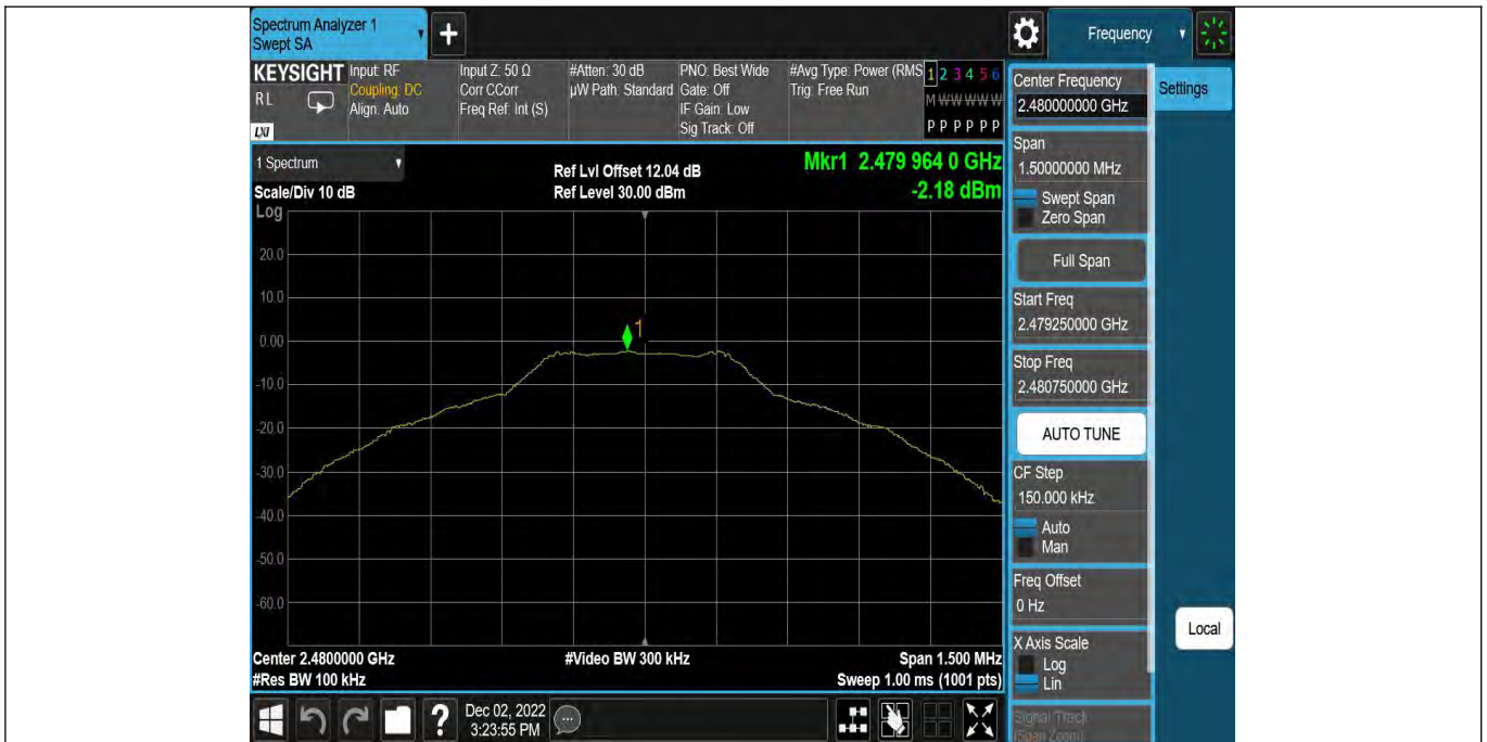
DH5-Ant1-2480-0~Reference--2.18
