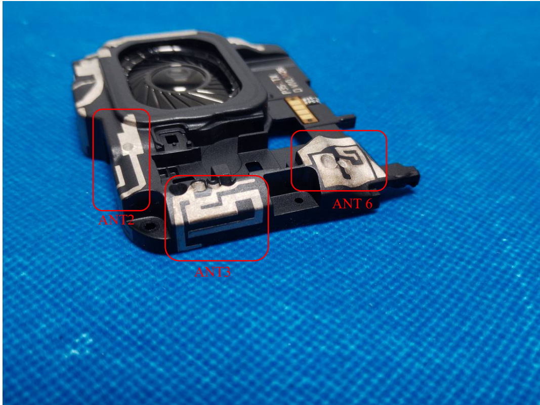
ANT2: Wi-Fi Chain1 ANT3: Wi-Fi Chain0/BT ANT6: 5G NR n7 DRX MIMO, n41 DRX
