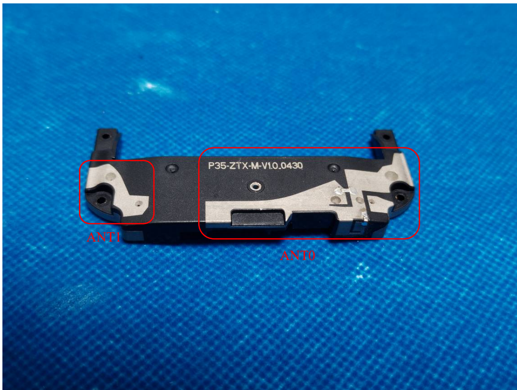
ANT0: GSM850/PCS1900, WCDMA B2/B4/B5, LTE B2/4/5/7/12/13/17/26/38/40/41/66, 5G NR n2/5/7/26/38/66 TRX ANT1: 5G NR n7 PRX MIMO, n41 TRX
