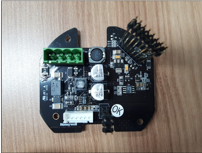
Top view of Host(Sub board)
