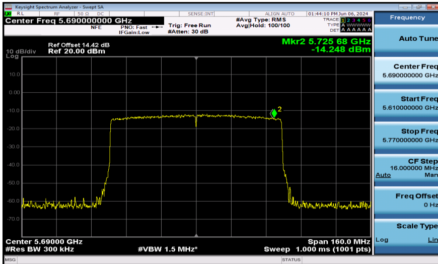
11AX80SISO-Ant1-5690_UNII-3-PASS
