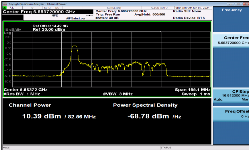
11AX80SISO-Ant1-5690_UNII-2C-52Tone-PASS
