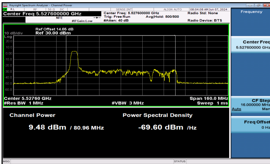
11AX80SISO-Ant1-5530-52Tone-PASS
