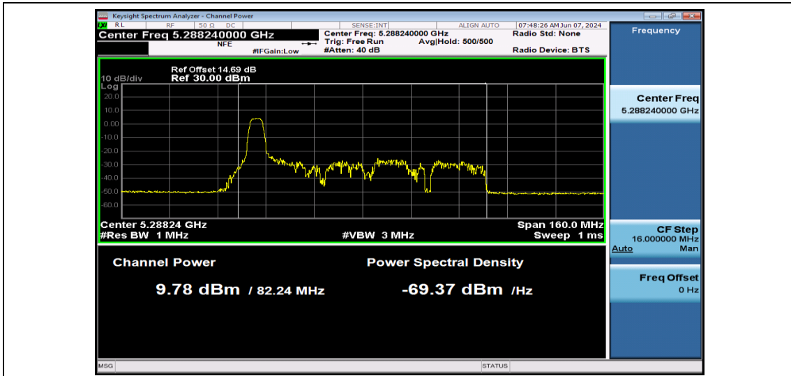
11AX80SISO-Ant1-5290-52Tone-PASS
