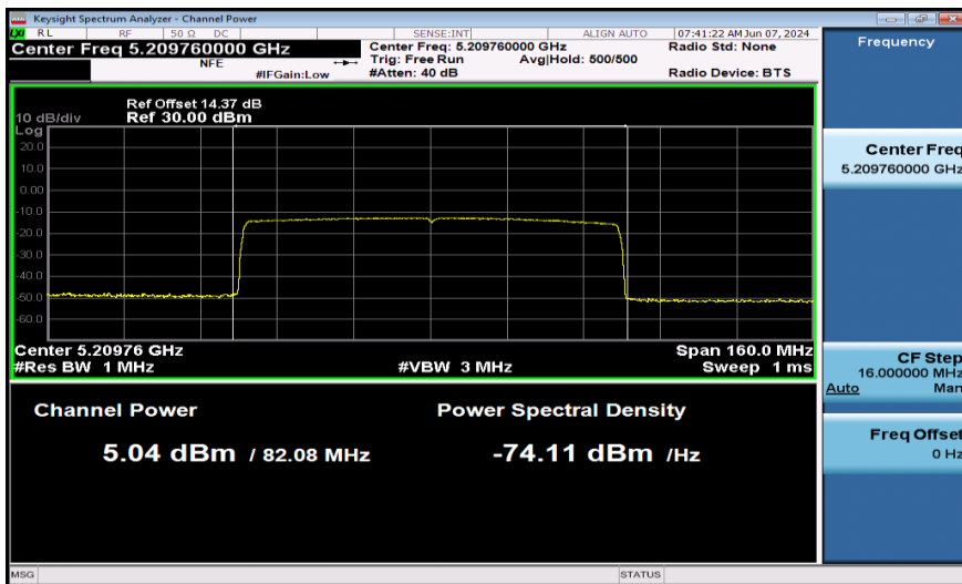
11AX80SISO-Ant1-5210-996Tone-PASS
