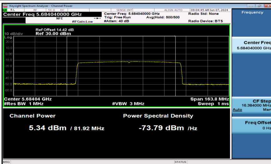
11AX80SISO-Ant1-5690_UNII-2C-996Tone-PASS
