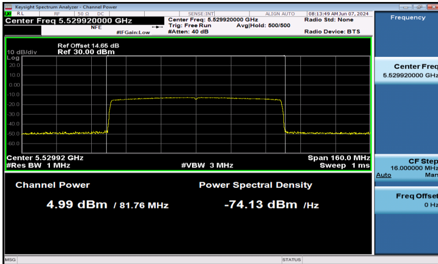
11AX80SISO-Ant1-5530-996Tone-PASS
