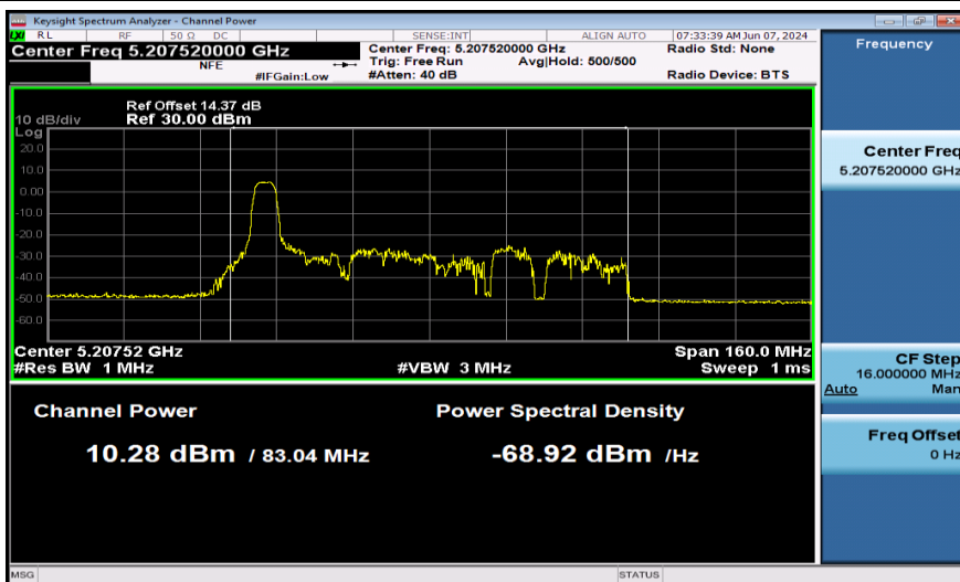
11AX80SISO-Ant1-5210-52Tone-PASS
