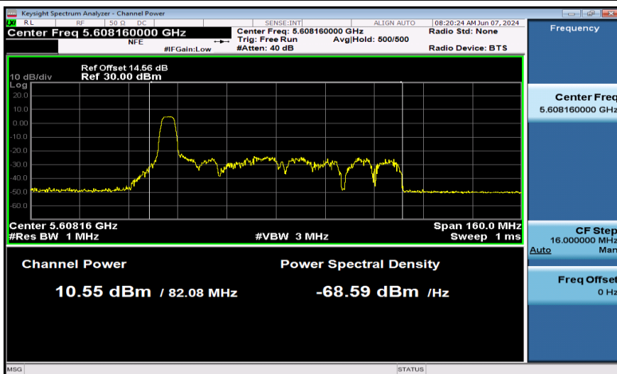
11AX80SISO-Ant1-5610-52Tone-PASS
