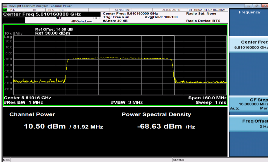
11AX80SISO-Ant1-5610-PASS
