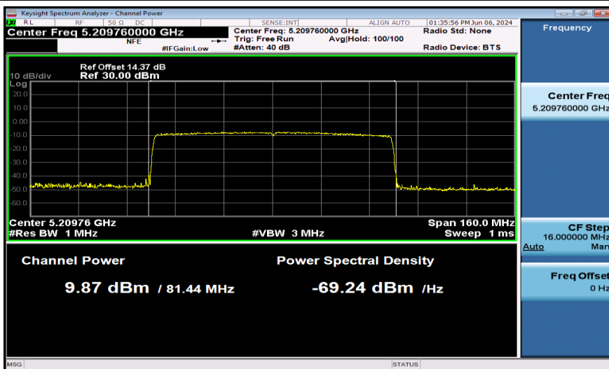
11AX80SISO-Ant1-5210-PASS
