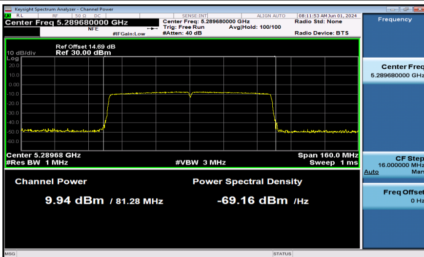
11AC80SISO-Ant1-5290-PASS
