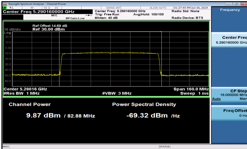
11AX80SISO-Ant1-5290-PASS
