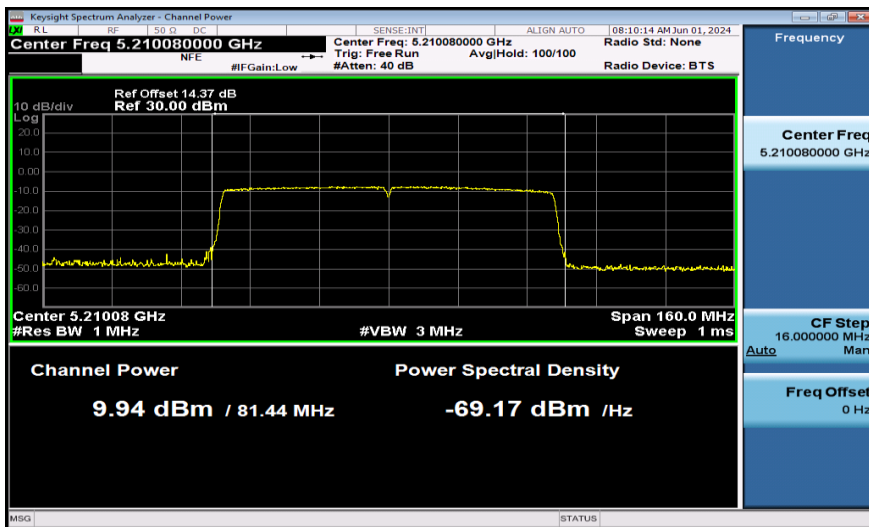
11AC80SISO-Ant1-5210-PASS
