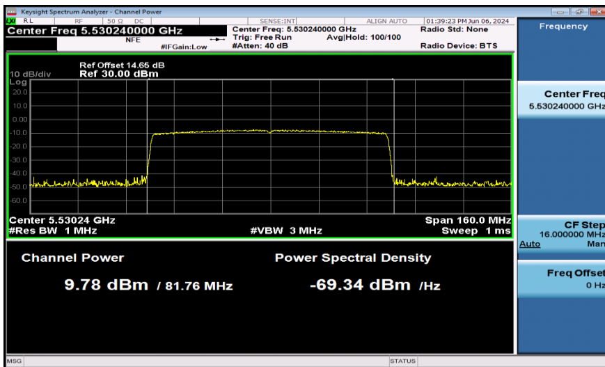
11AX80SISO-Ant1-5530-PASS
