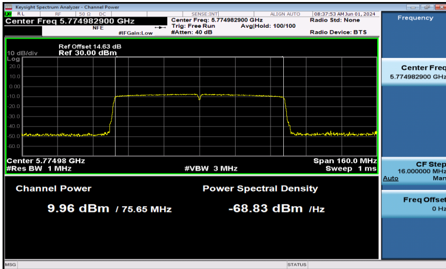
11AC80SISO-Ant1-5775-PASS
