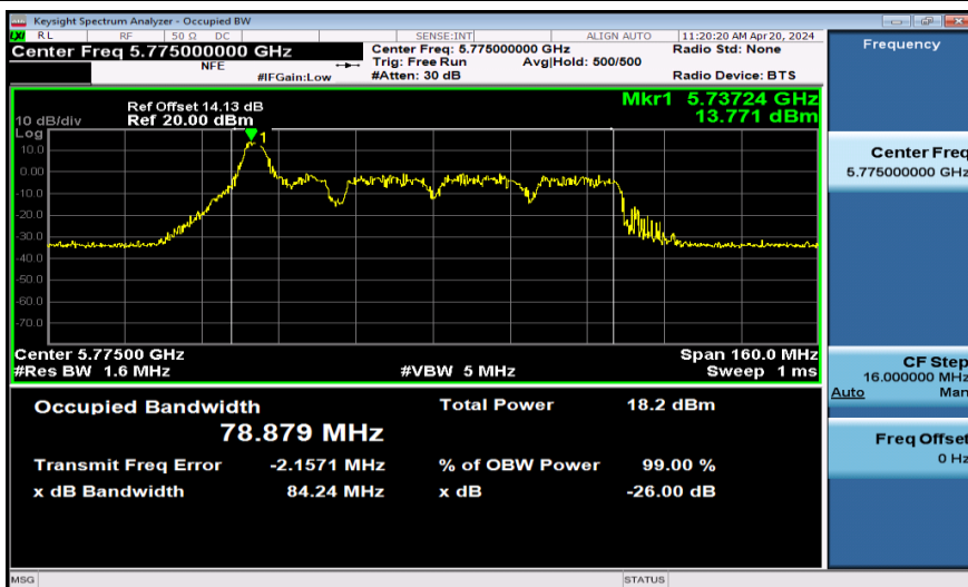
11AX80SISO-Ant1-5775-52Tone
