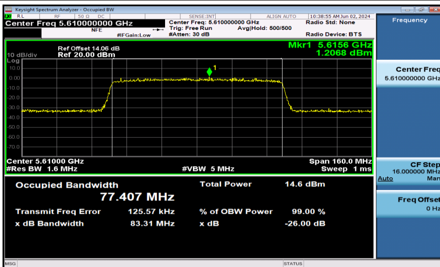
11AX80SISO-Ant1-5610-996Tone
