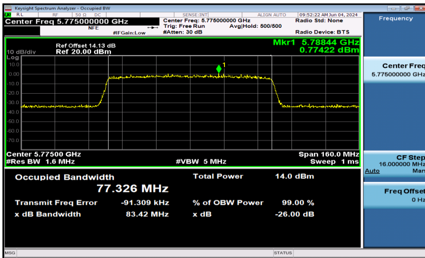
11AX80SISO-Ant1-5775-996Tone
