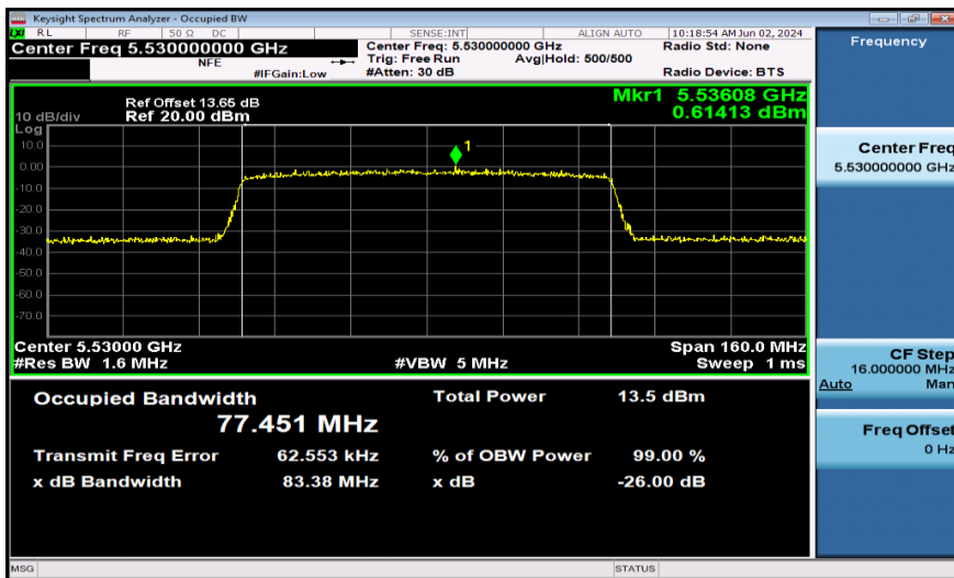
11AX80SISO-Ant1-5530-996Tone
