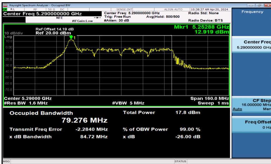
11AX80SISO-Ant1-5290-52Tone
