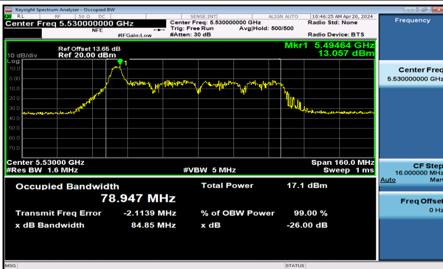
11AX80SISO-Ant1-5530-52Tone
