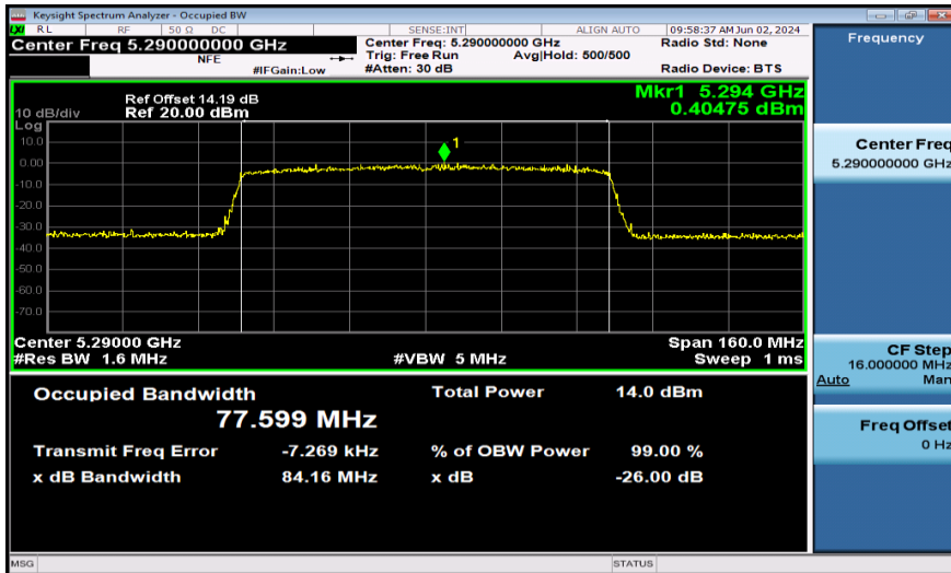
11AX80SISO-Ant1-5290-996Tone
