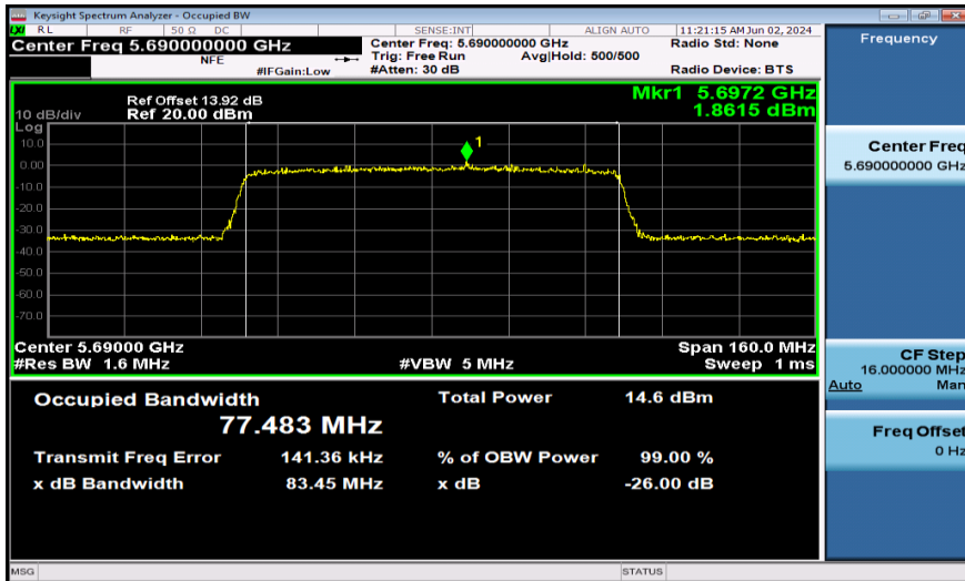
11AX80SISO-Ant1-5690-996Tone
