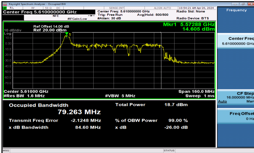
11AX80SISO-Ant1-5610-52Tone
