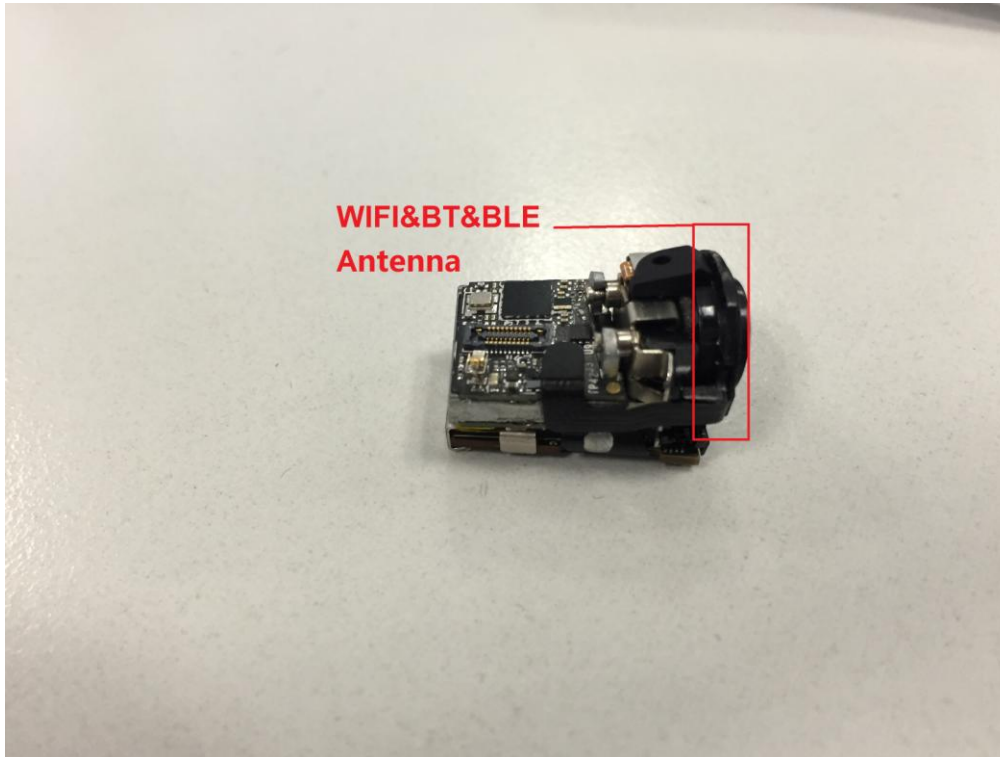
(20) EUT Photo
