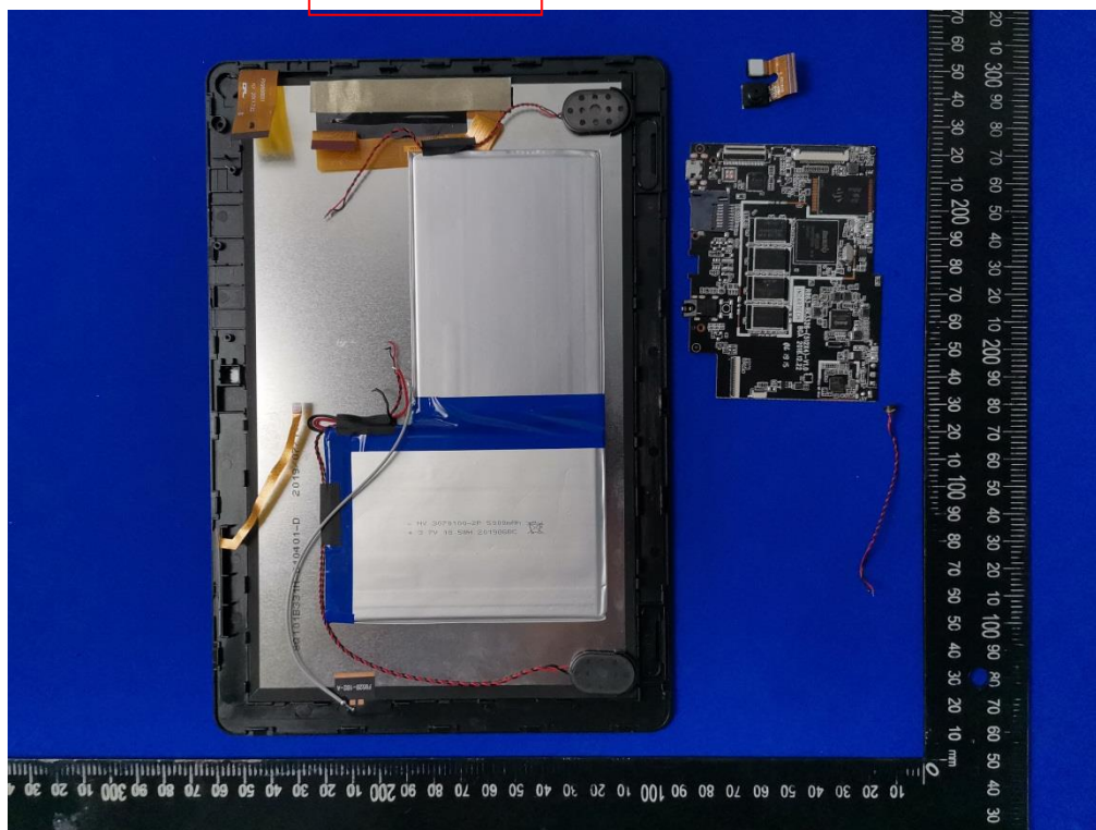
BT&WIFI Antenna
