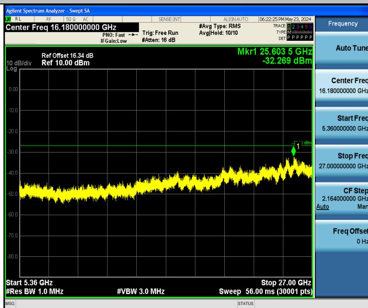
11A-Ant1-5200-5360~27000-PASS
