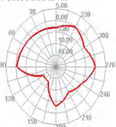
5750.000MHz E2
