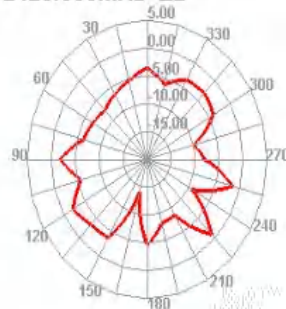
2425.000MHz E2
