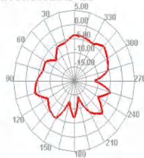
2500.000MHz E2
