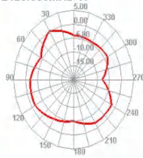
2425.000MHz H
