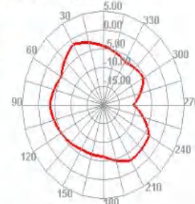
2450.000MHz E2
