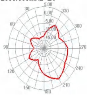
2500.000MHz E1
