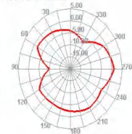
5350.000MHz E2
