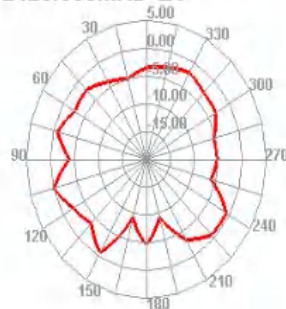
2425.000MHz E1
