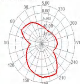
5850.000MHz H
