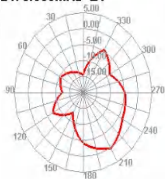
2475.000MHz E1
