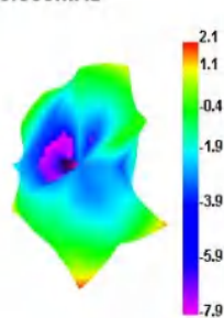
5550.000MHz
