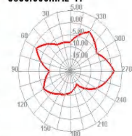
5350.000MHz E2
