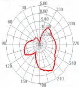
2425.000MHz E1
