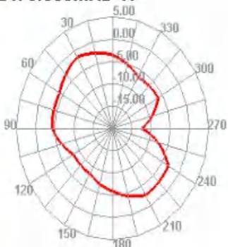
2475.000MHz H
