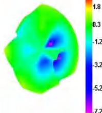
5850.000MHz E1
