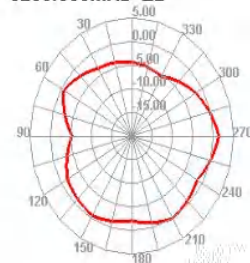
5250.000MHz E2
