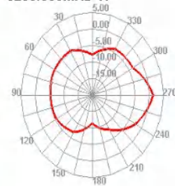
5250.000MHz H
