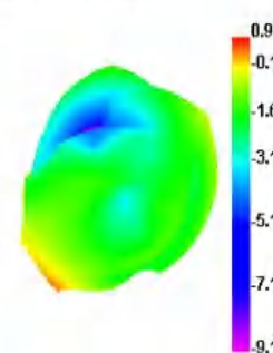
2450.000MHz E1
