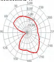
5550.000MHz H
