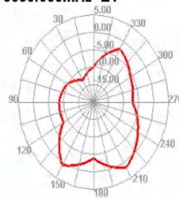
5350.000MHz E1
