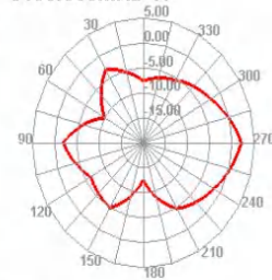
5150.000MHz E2
