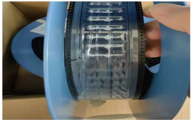
图2: 装箱包装方式
