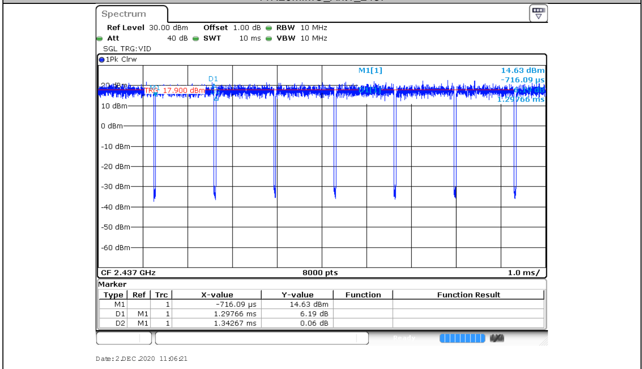
11N20MIMO_Ant2_2437
