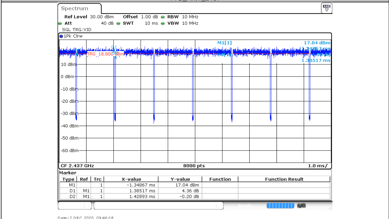
11G_Ant1_2437
