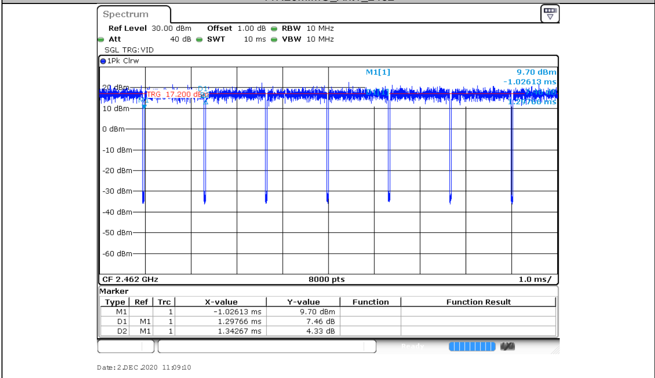
11N20MIMO_Ant2_2462
