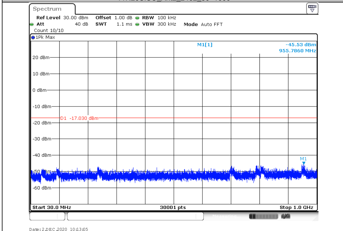
11N20SISO_Ant2_2462_30~1000
