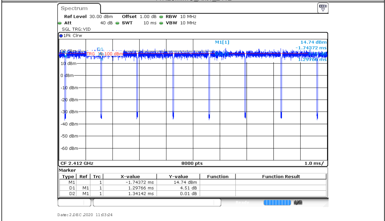
11N20MIMO_Ant2_2412
