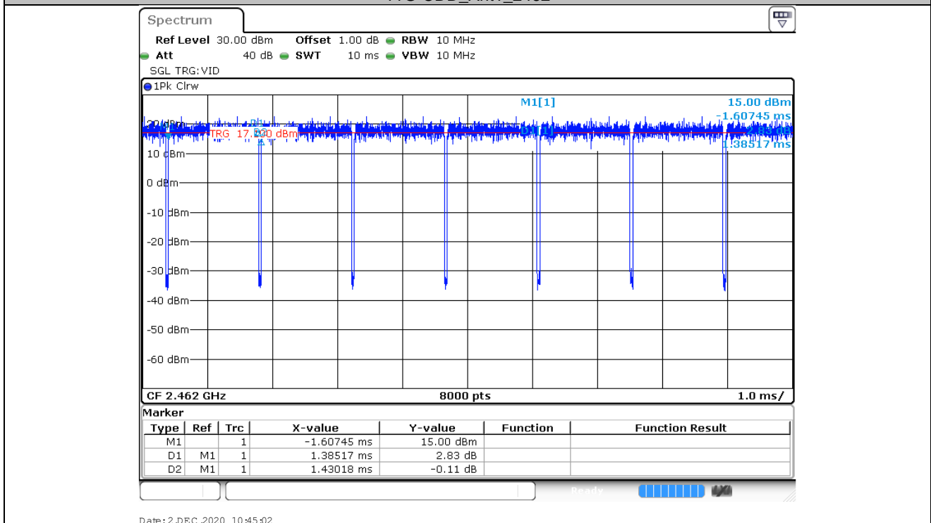
11G-CDD_Ant1_2462
