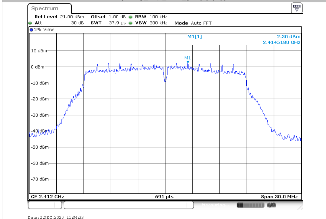
11N20MIMO_Ant1_2412_0-Reference
