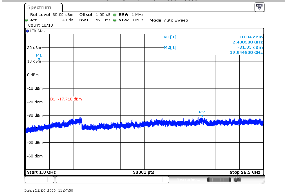
11N20MIMO_Ant2_2437_0~Reference
