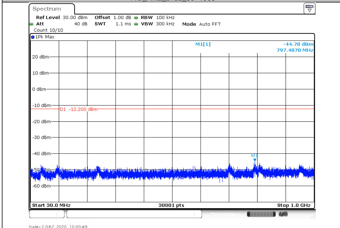
11B_Ant2_2462_30~1000
