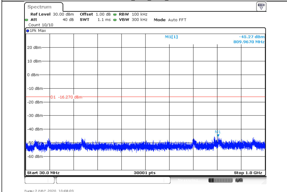
11N20SISO_Ant2_2412_30~1000
