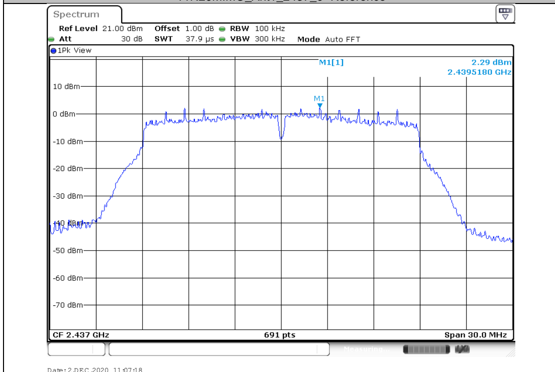
11N20MIMO_Ant1_2437_0-Reference
