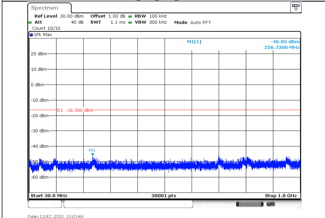
11G_Ant2_2462_30~1000
