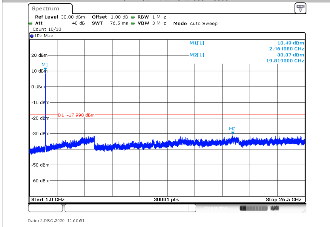
11N20MIMO_Ant2_2462_0~Reference
