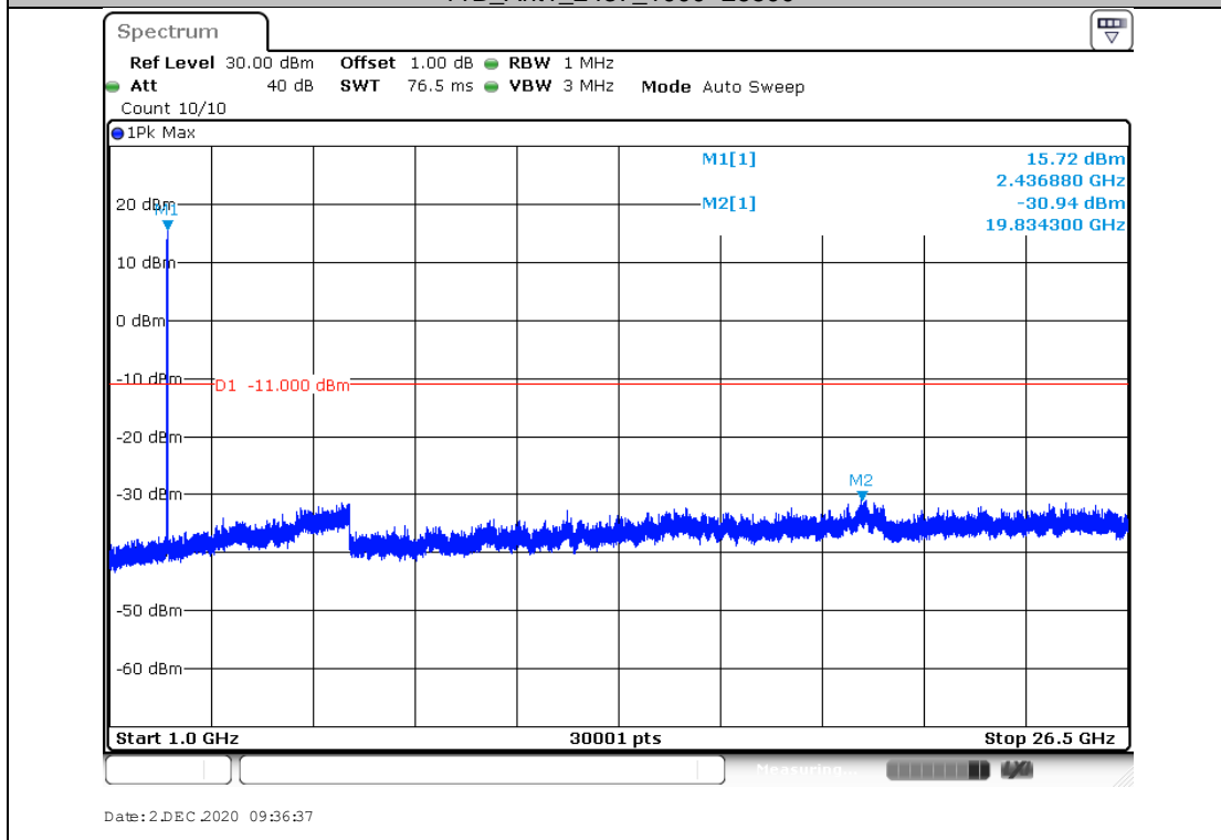
11B_Ant2_2437_0~Reference
