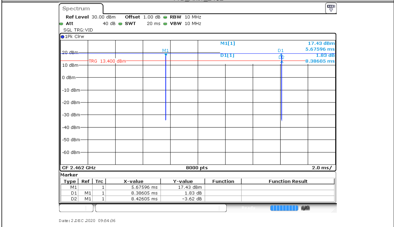
11B_Ant2_2462
