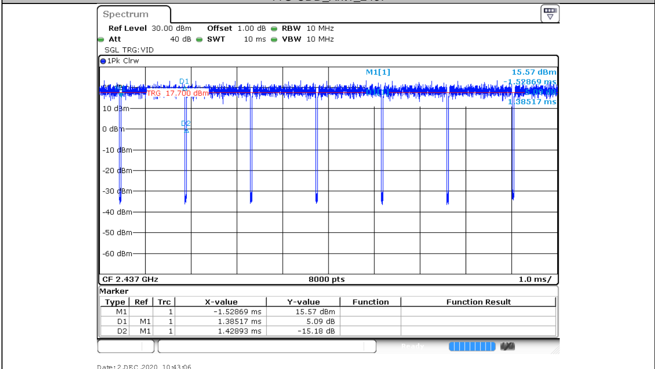
11G-CDD_Ant1_2437
