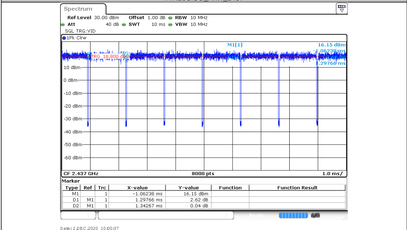
11N20SISO_Ant1_2437
