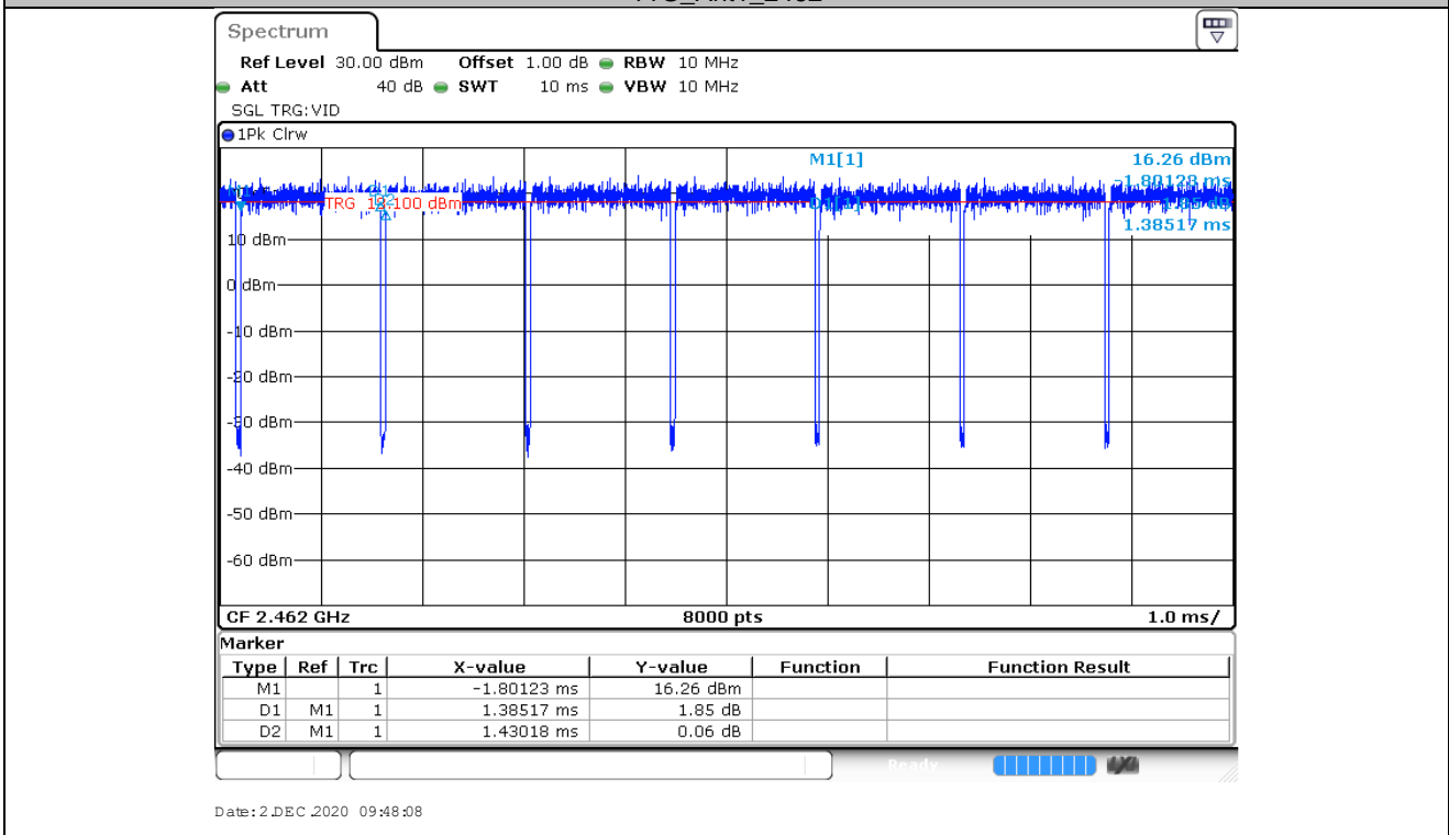
11G_Ant2_2462
