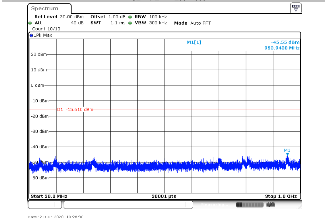
11G_Ant2_2412_30~1000
