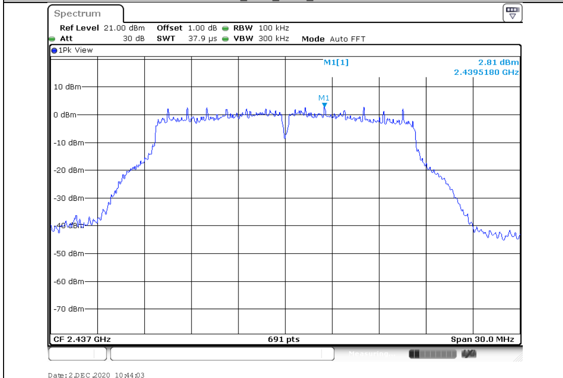
11G-CDD_Ant1_2437_0-Reference
