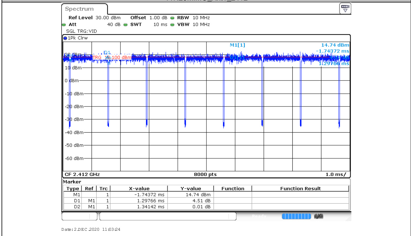
11N20MIMO_Ant2_2412
