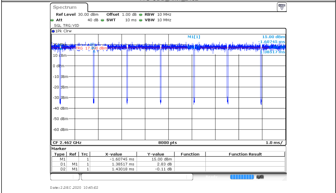
11G-CDD_Ant2_2462
