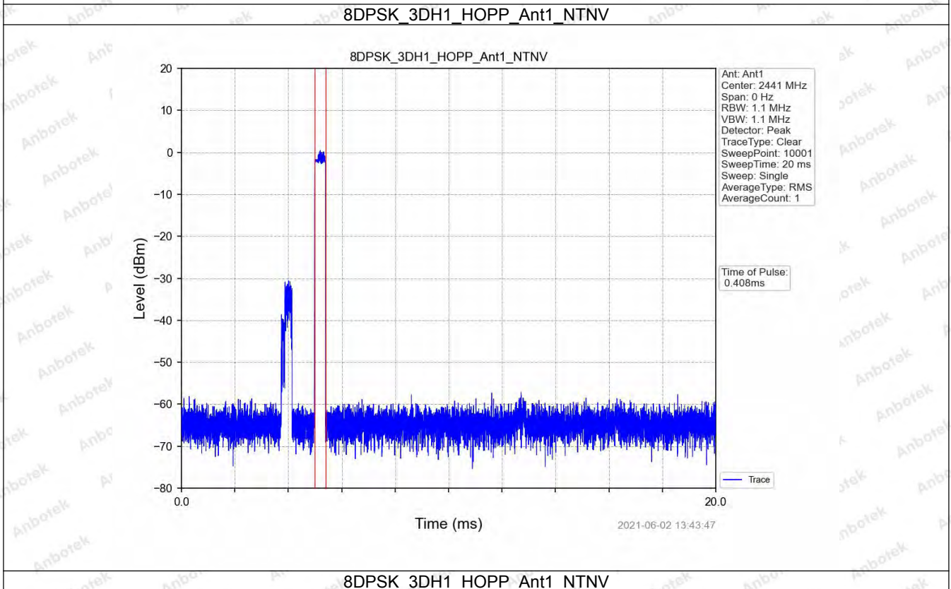
8DPSK_3DH1_HOPP_Ant1_NTNV
