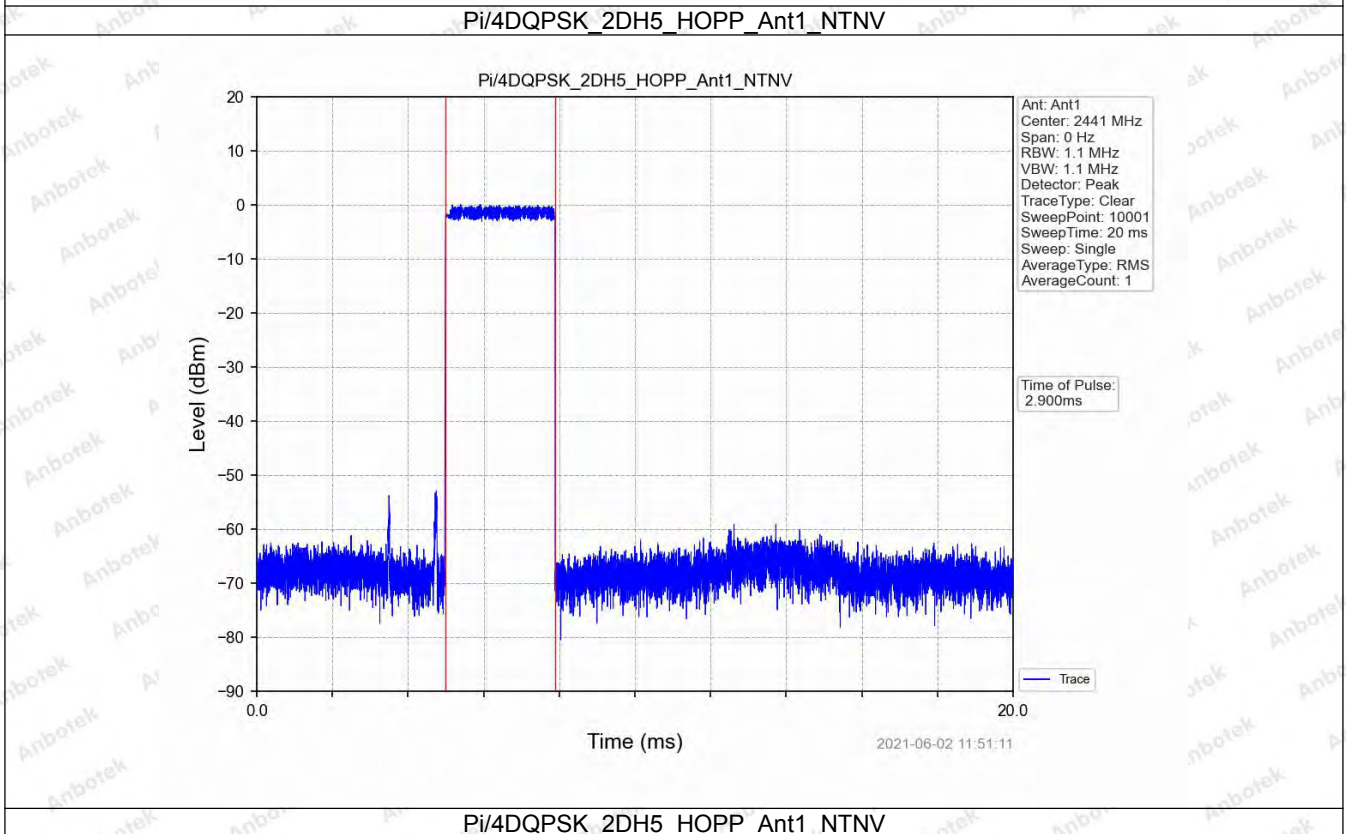
Pi/4DQPSK_2DH5_HOPP_Ant1_NTNV
