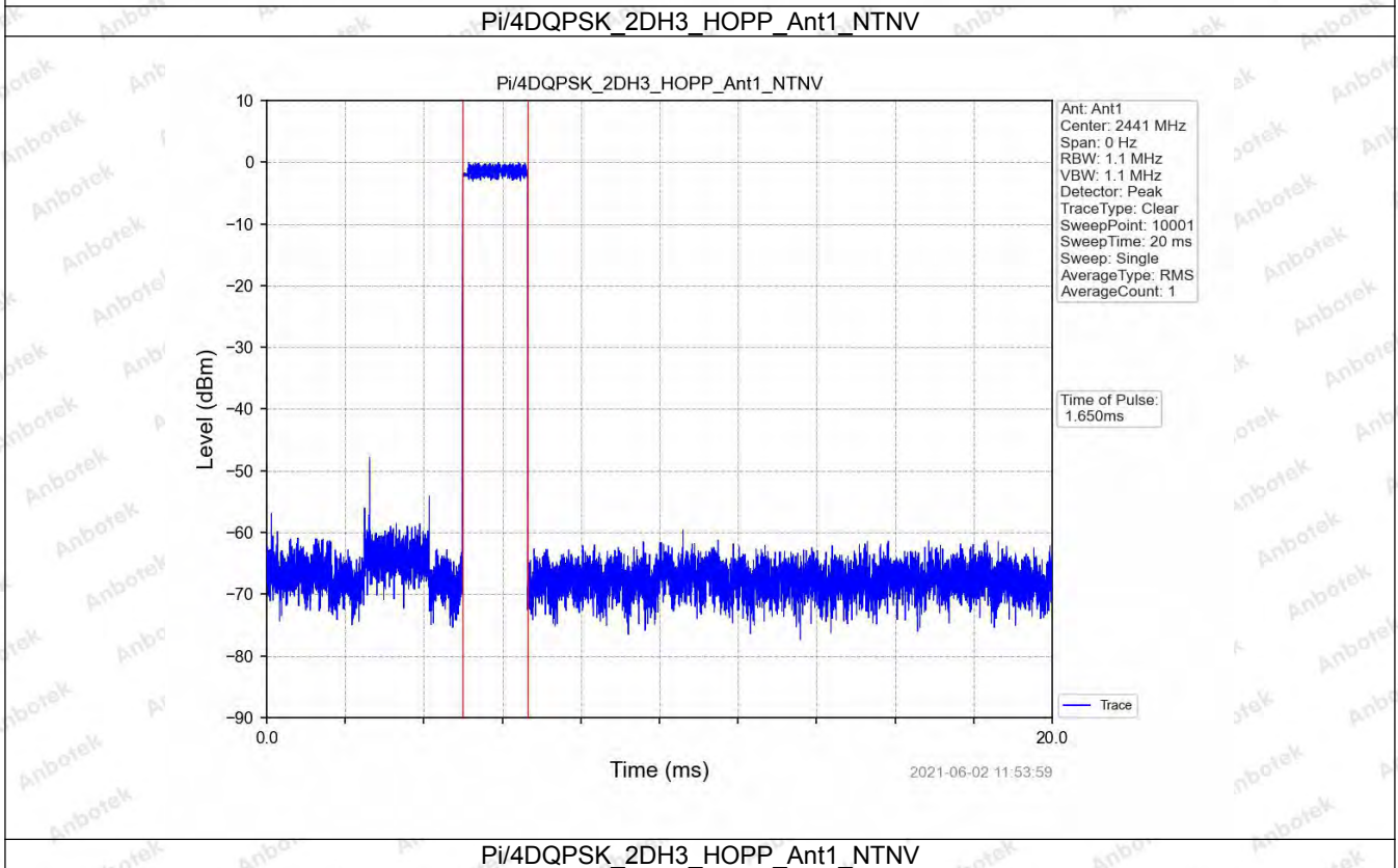
Pi/4DQPSK_2DH3_HOPP_Ant1_NTNV
