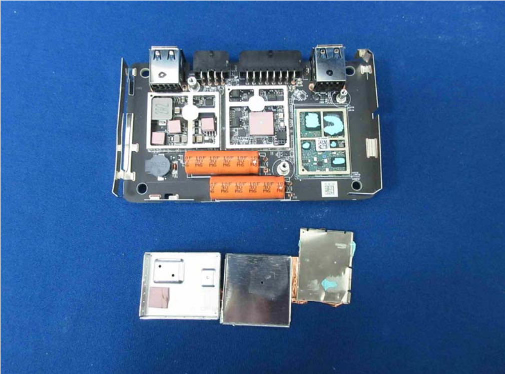
(16) EUT Photo
