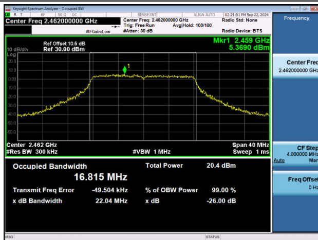
11G-Ant1-2462
