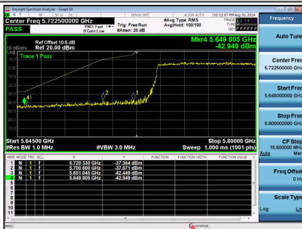
11AX80SISO-Ant2-5775-PASS
