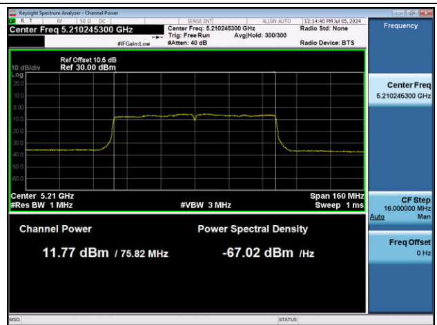
11AC80SISO-Ant1-5210-PASS
