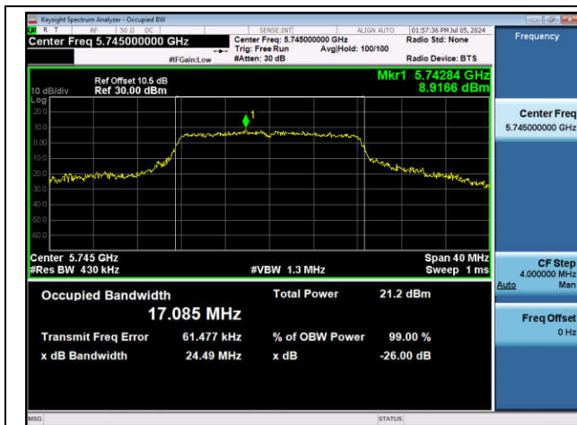
11A-Ant1-5745
