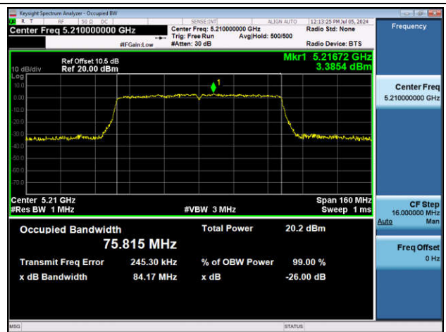
11AC80SISO-Ant1-5210
