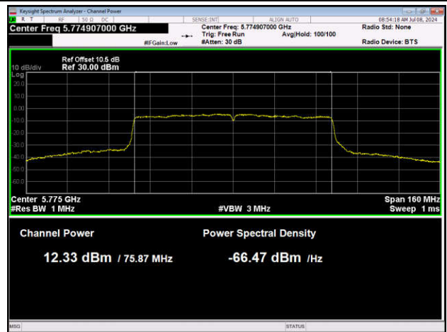
11AC80SISO-Ant1-5775-PASS
