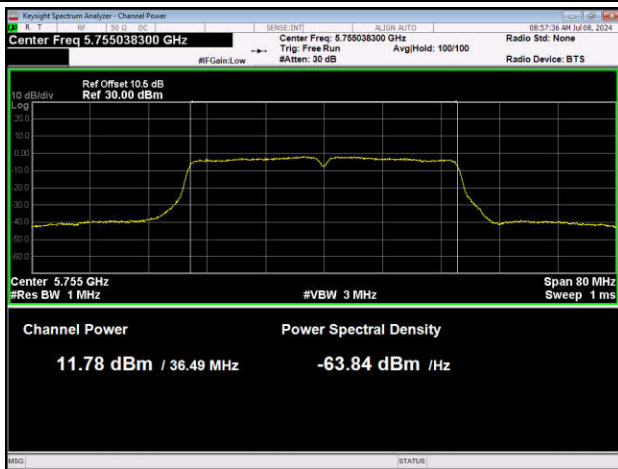
11N40SISO-Ant1-5755-PASS
