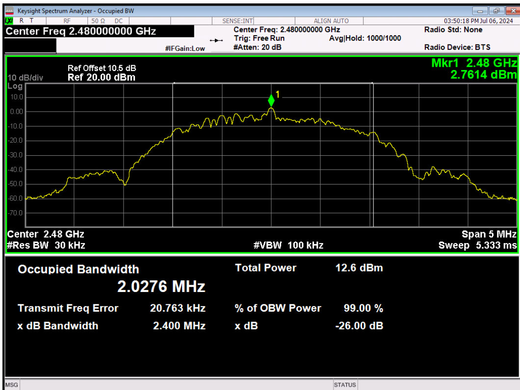
BLE_2M-Ant1-2480
