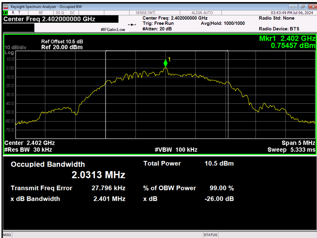
BLE_2M-Ant1-2402
