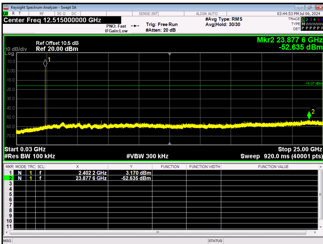
BLE_2M-Ant1-2402-30~25000-PASS
