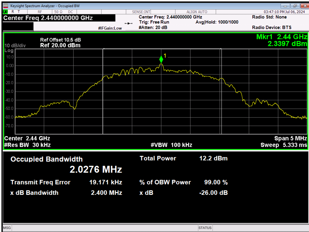
BLE_2M-Ant1-2440
