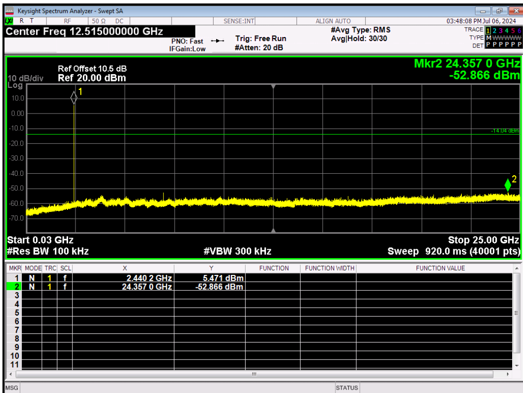
BLE_2M-Ant1-2440-30~25000-PASS
