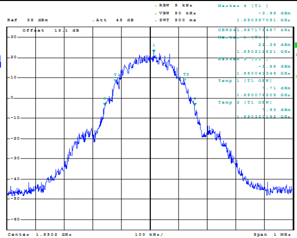
GPRS1900
