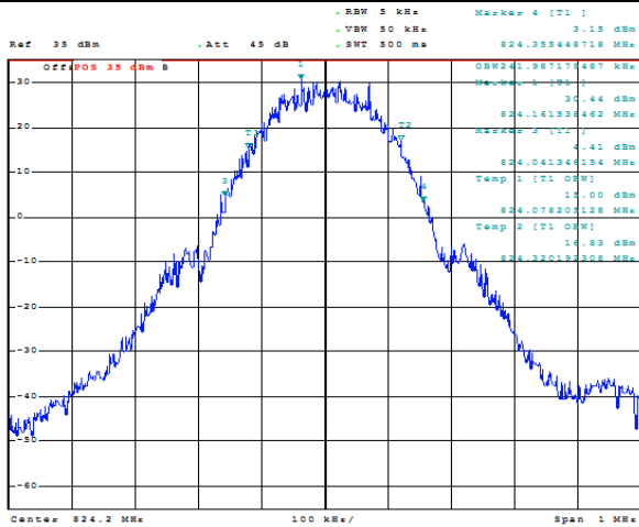
GPRS 850
