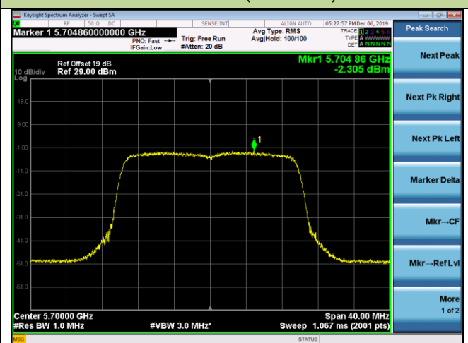
Channel 140 (5700MHz)
