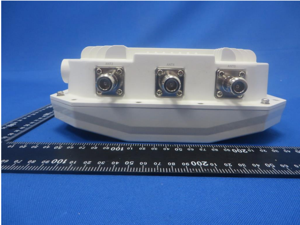
(19) EUT Photo - OAW-AP1362
