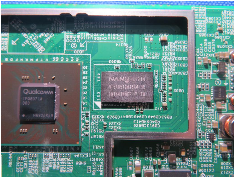
(5) EUT Photo_OAW-AP1321
