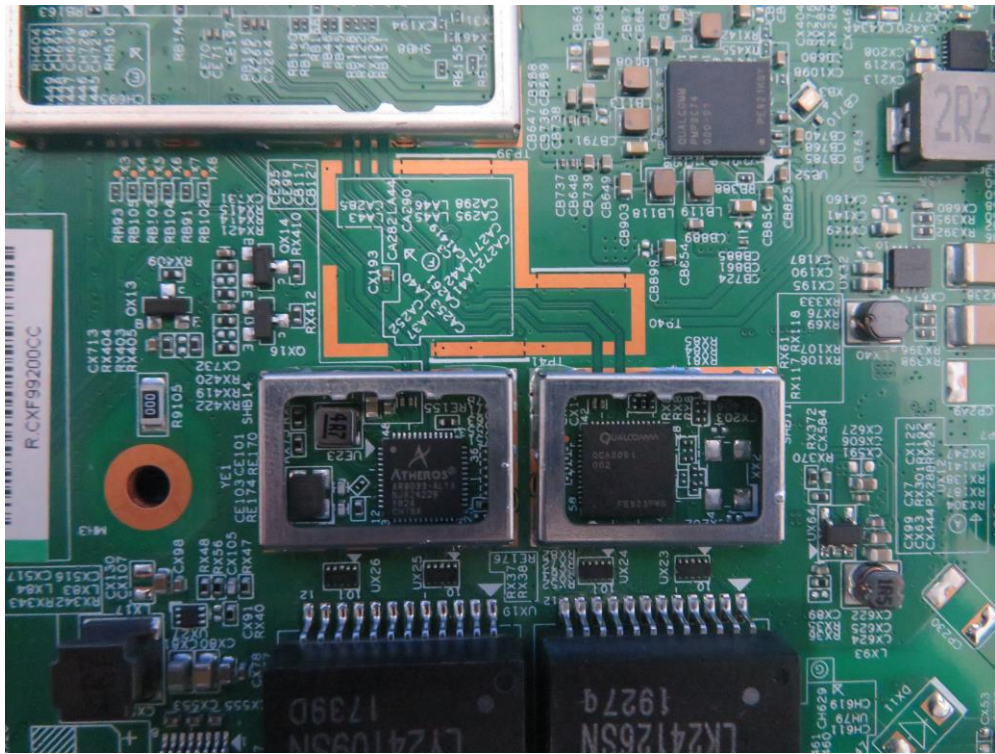
(7) EUT Photo_OAW-AP1321
