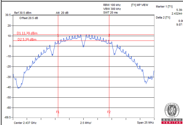
802.11n (20MHz) / Chain 0: CH6
