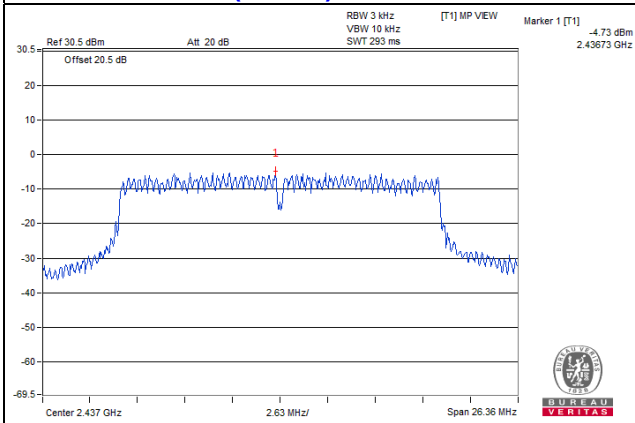
802.11n (20MHz) / Chain 3: CH6
