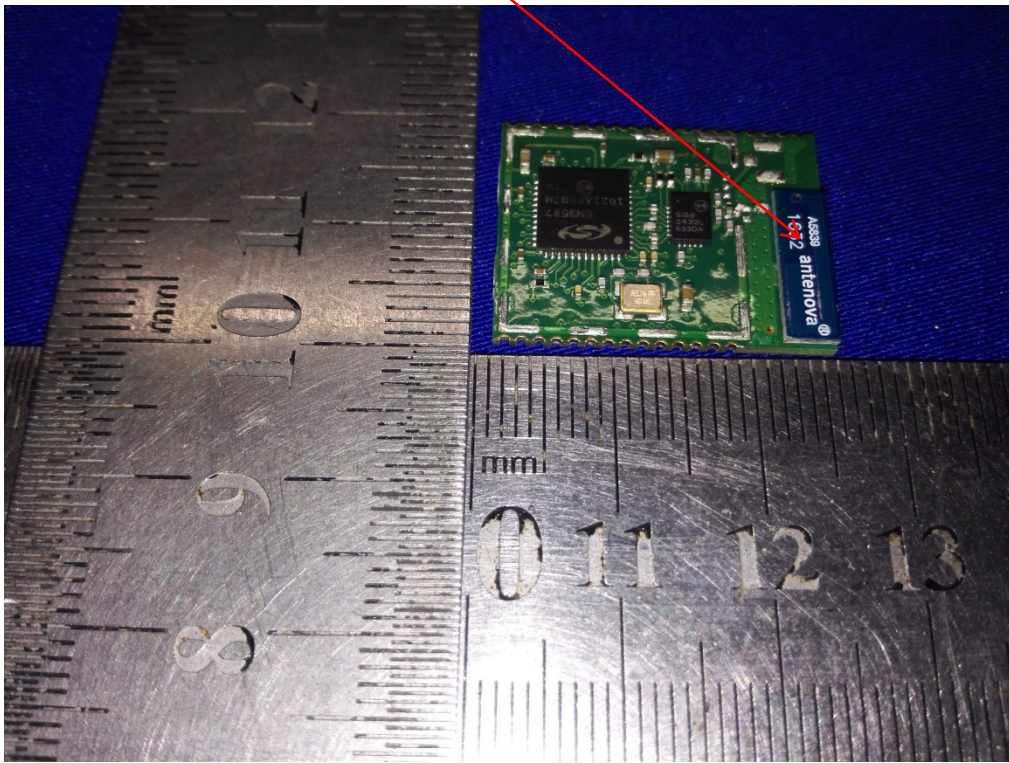
Zigbee Module
