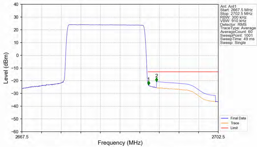
41_Single_NTNV_CC1:15MHz_QPSK_CC1:2682.5MHz_Ant1
