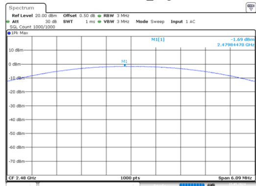
\pi/4 -DQPSK_High
