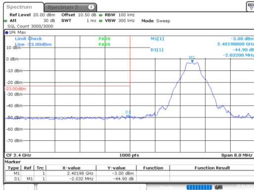
GFSK_Low_DH1
