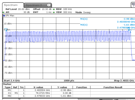
GFSK_Hopping_DH1
