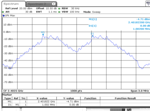
GFSK_Low_DH1
