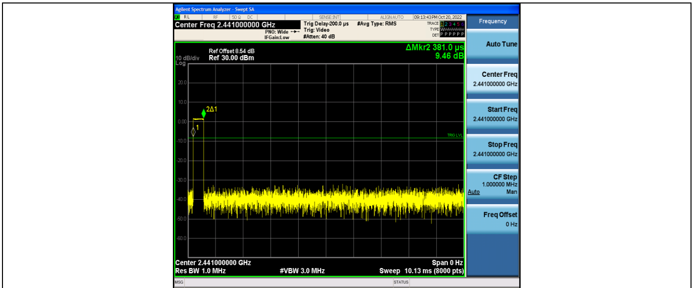
DH1_Ant1_Hop
