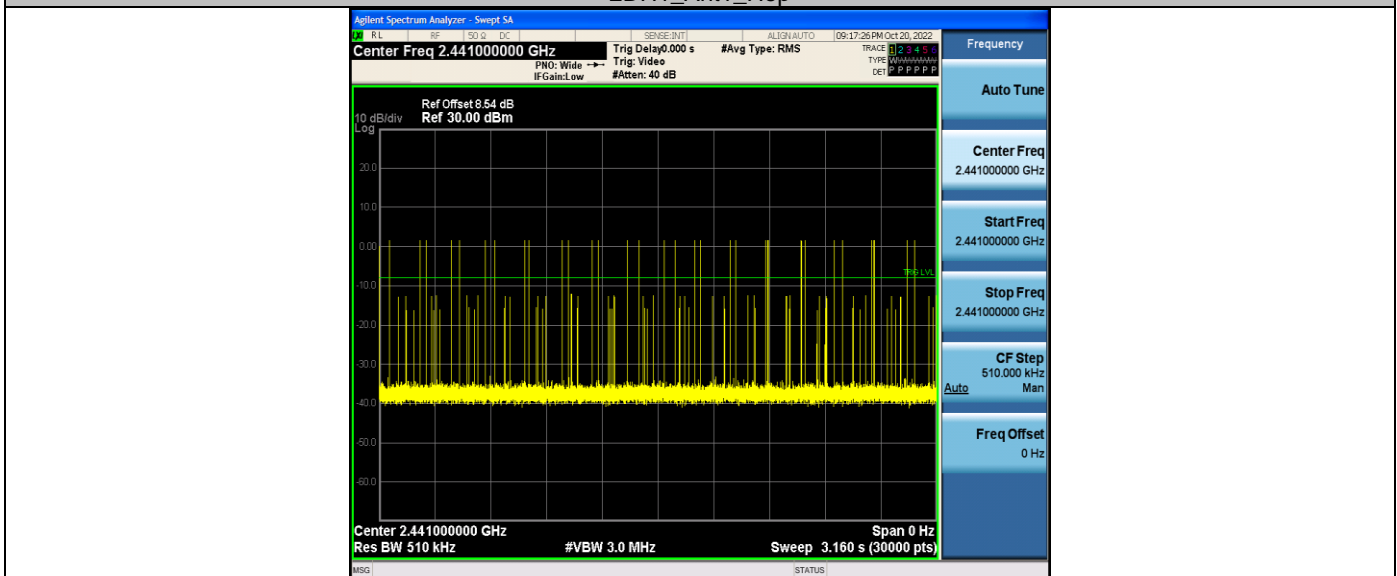
2DH1_Ant1_Hop
