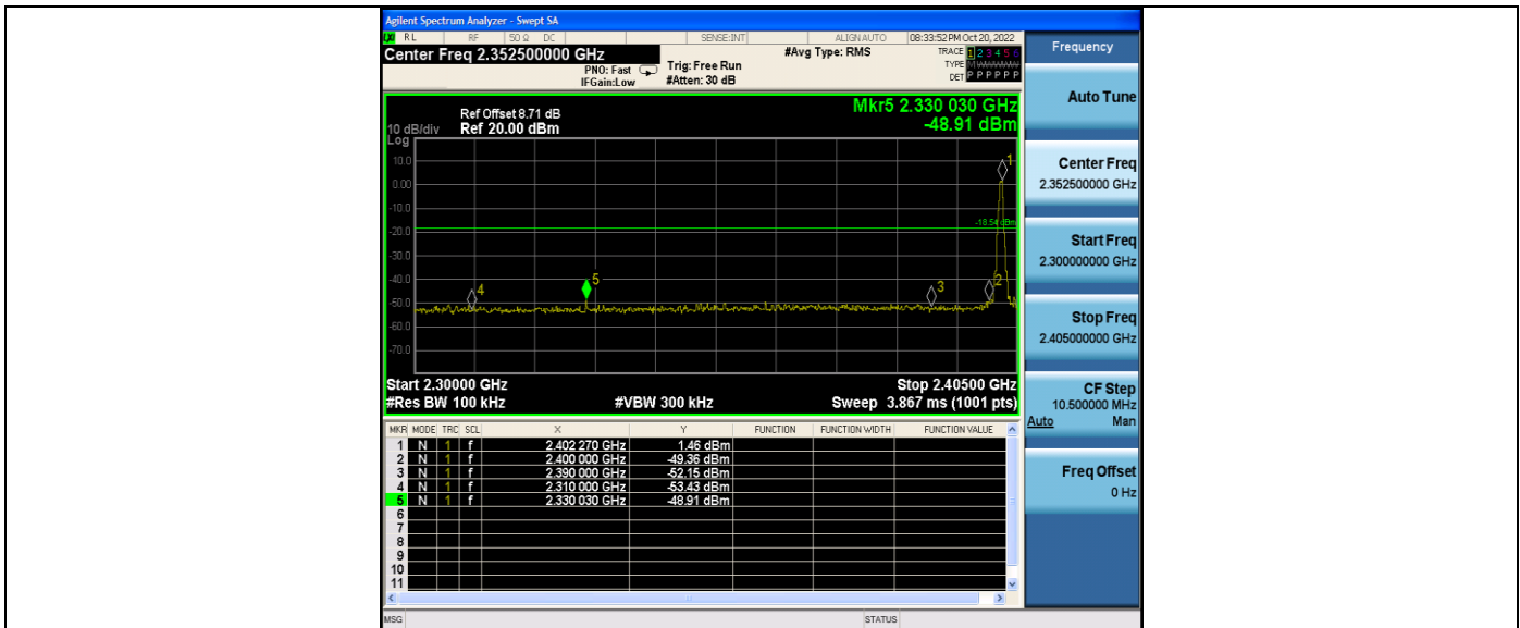
DH5_Ant1_Low_2402
