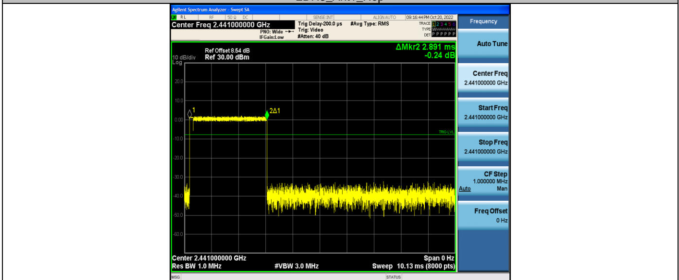
2DH5_Ant1_Hop
