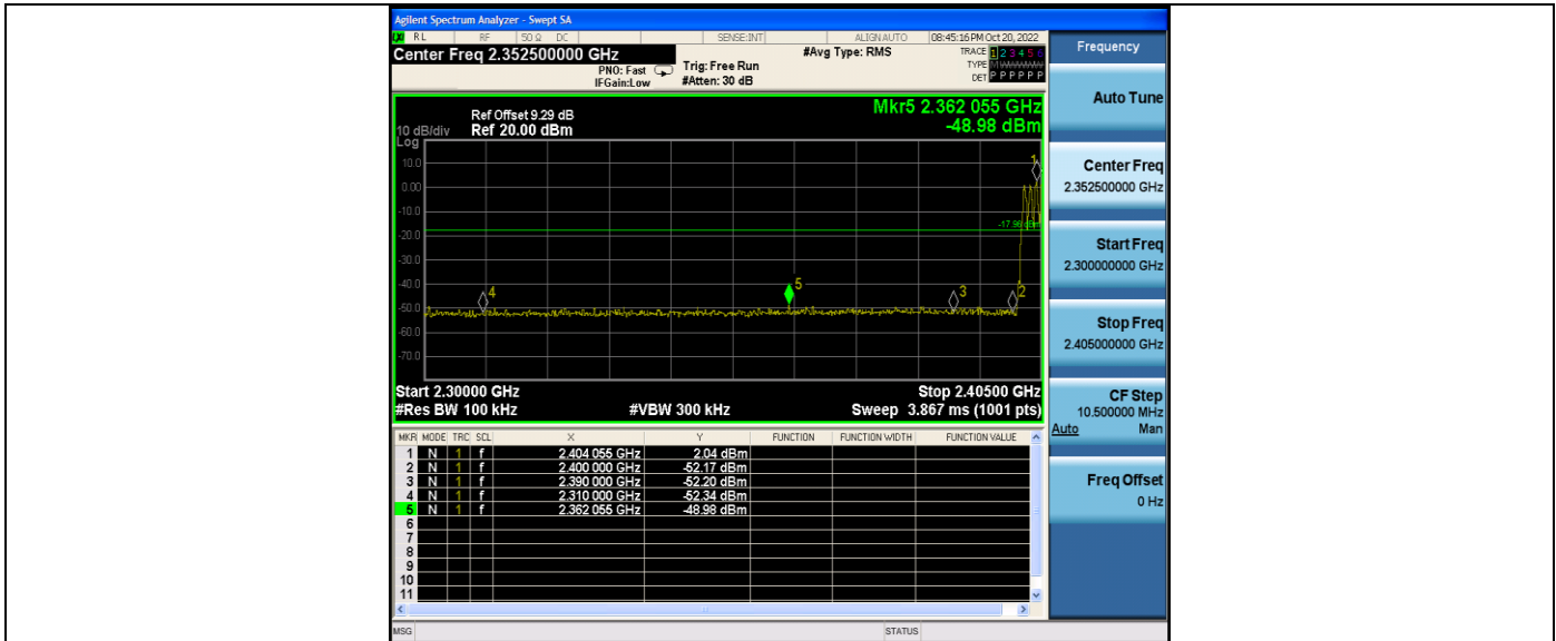
DH5_Ant1_Low_Hop_2402
