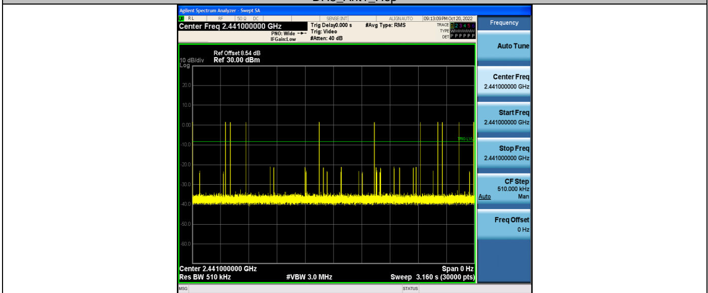
DH5_Ant1_Hop
