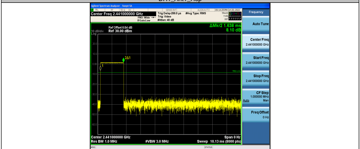
DH3_Ant1_Hop
