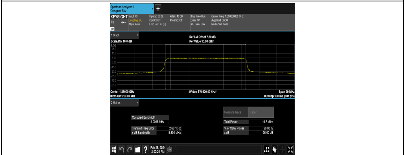
Band2-10MHz-QPSK-18900-50RB#0
